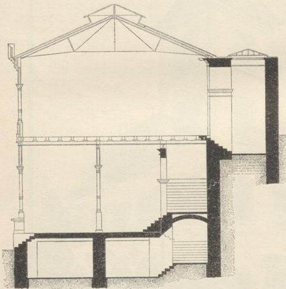
Fig. 361. Querschnitt.
