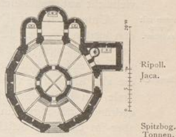
Fig. 547. Segovia, Tempelkirche. (Nach Street.)
