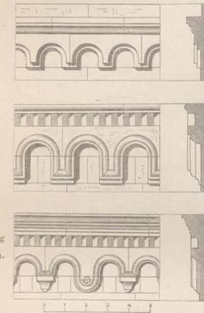
Fig. 412—414. Bogenfriese von der Kirche zu Schöngrabern. (Nach Heider.)
