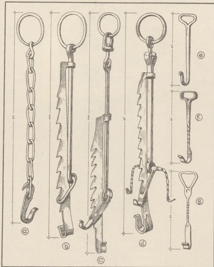
Abb. 55. Kesselhaken.
