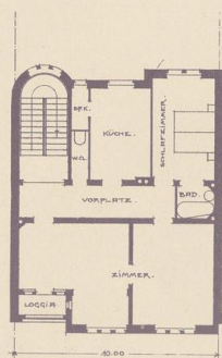
WOHNUNGSGESCHOSS.
