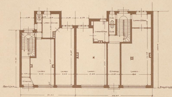
GRUNDRISS DES ERDGESCHOSSES.
