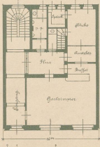
Erdeggeschoss
