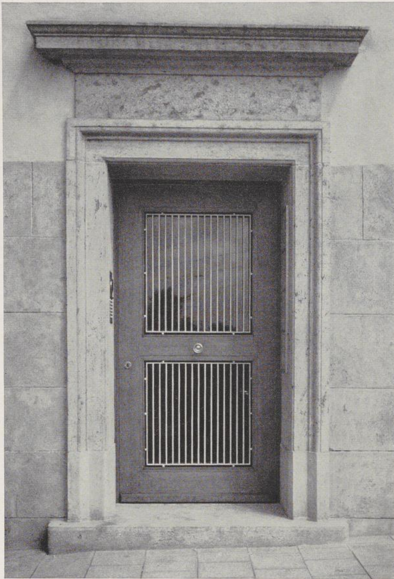
Seiteneingangs-Türe an einem Versicherungsgebäude, Holz Eisenstäbe weiß gestrichen, dahinter Klarglasscheibe, Messingknopf
