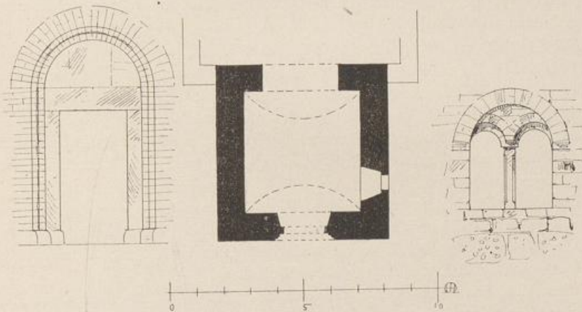
Fig. 85. Vochem. Kathol. Pfarrkirche, Nordansicht und Einzelheiten vom Turme.
