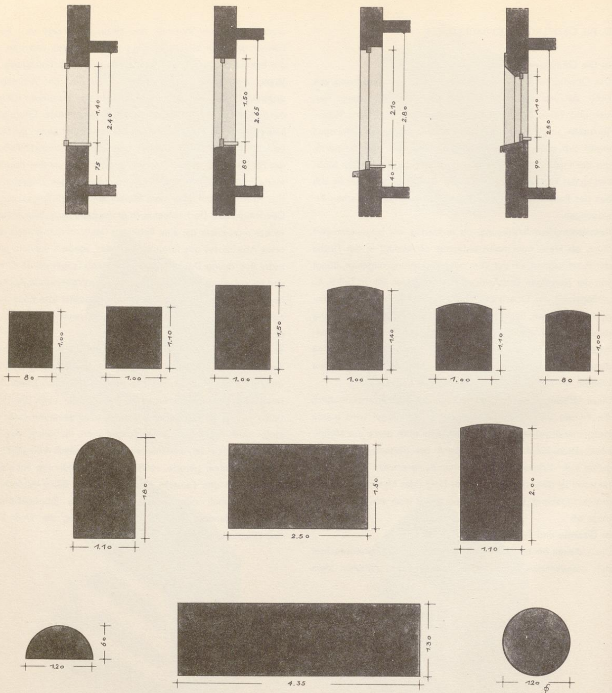
Fensteröffnungen. Oben in Vertikalschnitten. Die Fenster selbst in verschiedenen Größen und Formaten.
