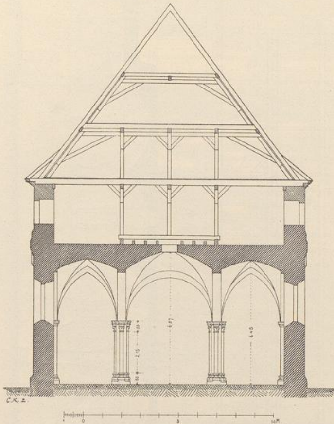
M. = 1:200 Fig. 145. Nieder-Weisel. Querschnitt der Johanniterkirche.
