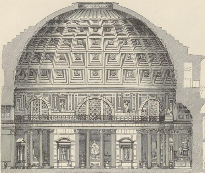
1. Pantheon in Rom, 27 v. Chr. von Agrippa gestiftet. (Durchschnitt.)
