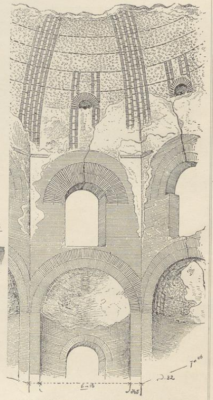
10. Kuppelkonstruktion des Zehncks der sogen. Minerva Medica in Rom. (Nach Durm.)
