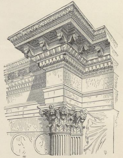
4. Gebälk vom Constantinsbogen. (Verkröpfung.)
