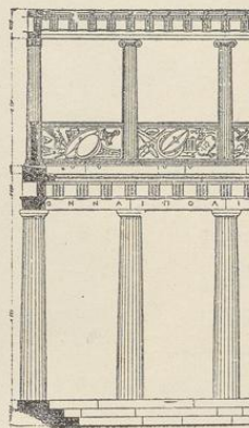
7. Griechenland. Zweistöckige Säulenhalle in Pergamon. (System nach Bohn.)
