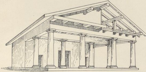
5. Etruskischer Tempel nach Vitruv. (Nach Borrmann und Wiegand.) (Giebel links mit verschaltem, rechts mit offenem Gebälk; alles Schmuckwerk ist fortgelassen.)
