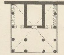
3. Etruskischer Tempel nach Vitruv.
