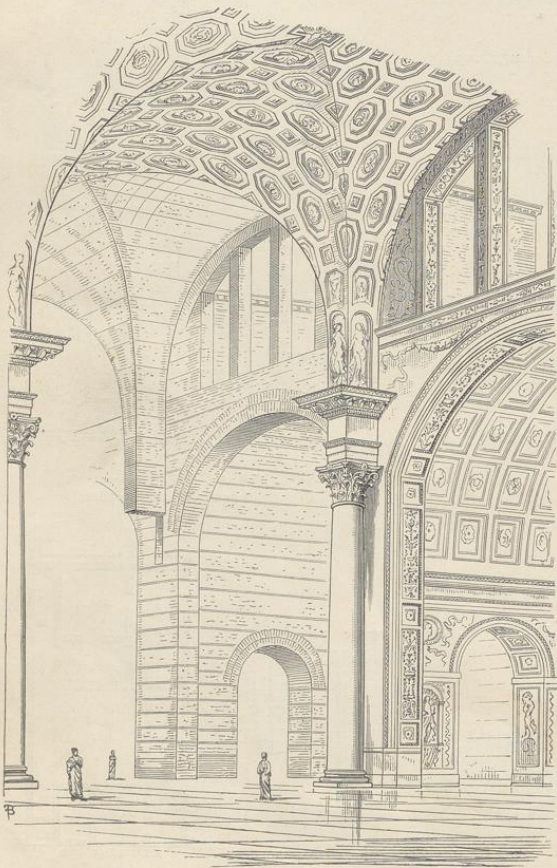
9. Gewölbesystem der Basilika des Maxentius in Rom.
