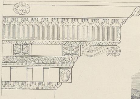
2. Gebälk vom Dioscurentempel in Rom.
