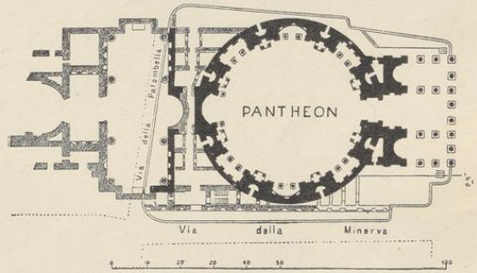
2. Grundriß des Pantheons. (Nach Durm.)
