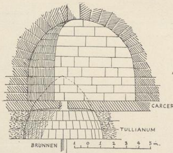
Querschnitt.
