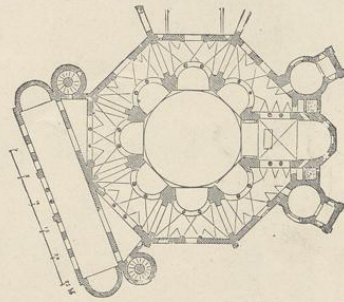
4. Grundriß von San Vitale in Ravenna.
