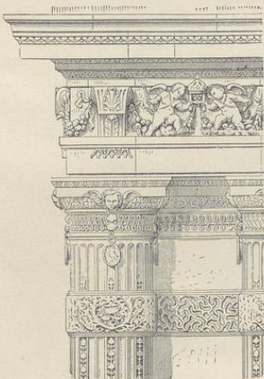
5. Säule von den Tuileries.
