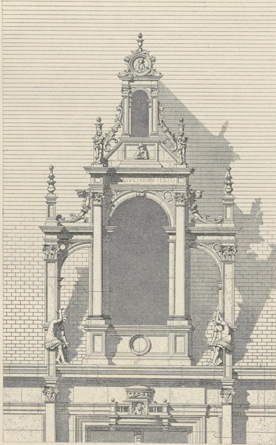
1. Lucarne vom Hotel Ecoville in Caen. (Um 1530.) (Nach Sauvageot.)
