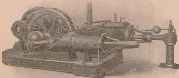
Luft-Kompressor für Elektro-Motor durch Zahnräder getrieben.
