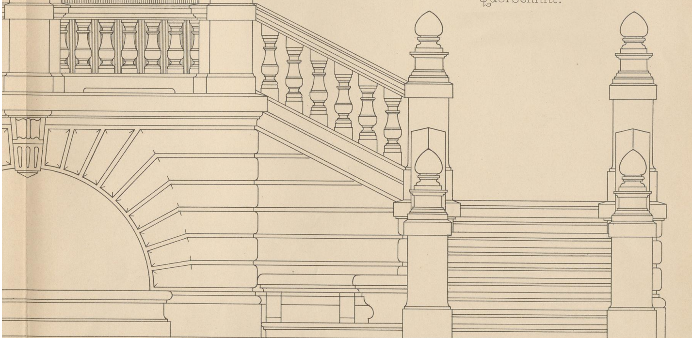
eransicht.
