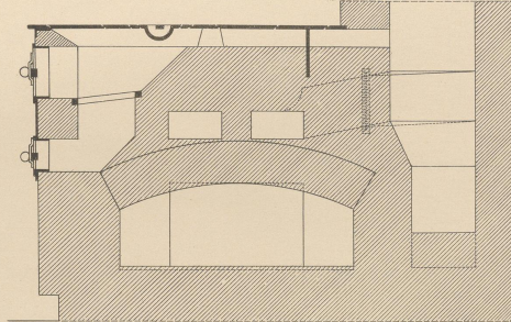
Längenschnitt.
