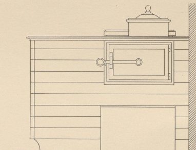
Seitenansicht.
