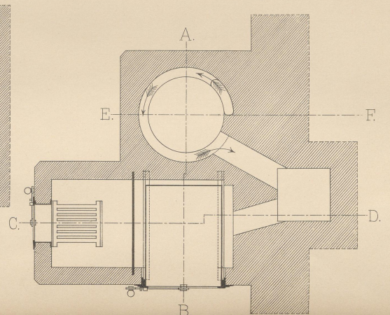
Grundriss.
