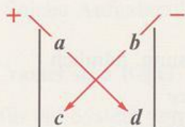
Abb. 140.1 Zur Berechnung einer zweireihigen Determinante
