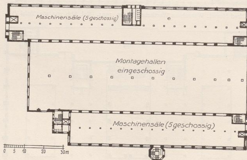
Peter Behrens: Fabriken der AEG, Berlin, Am Humboldtthain. 1909—1912. Plan der Gesamtanlage und Grundriß der Hochspannungsfabrik (Vgl. Abb. 294—298)
