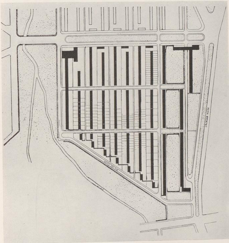
Walter Gropius: Siedlung Dammerstock, Karlsruhe. 1929
