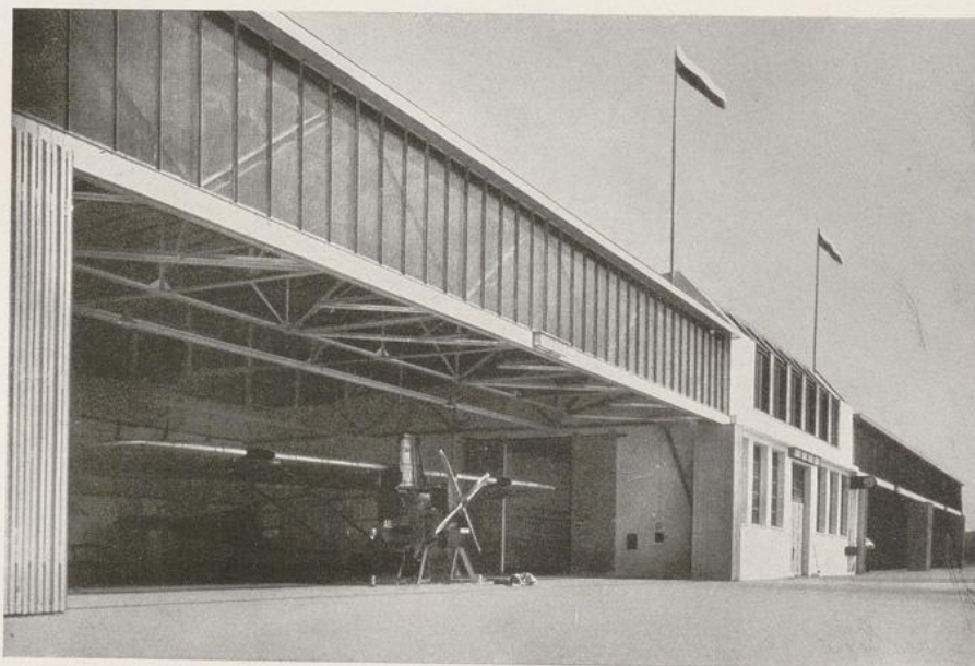
Heinrich Kosina: Flugzeughalle, Berlin-Tempelhof. 1926
