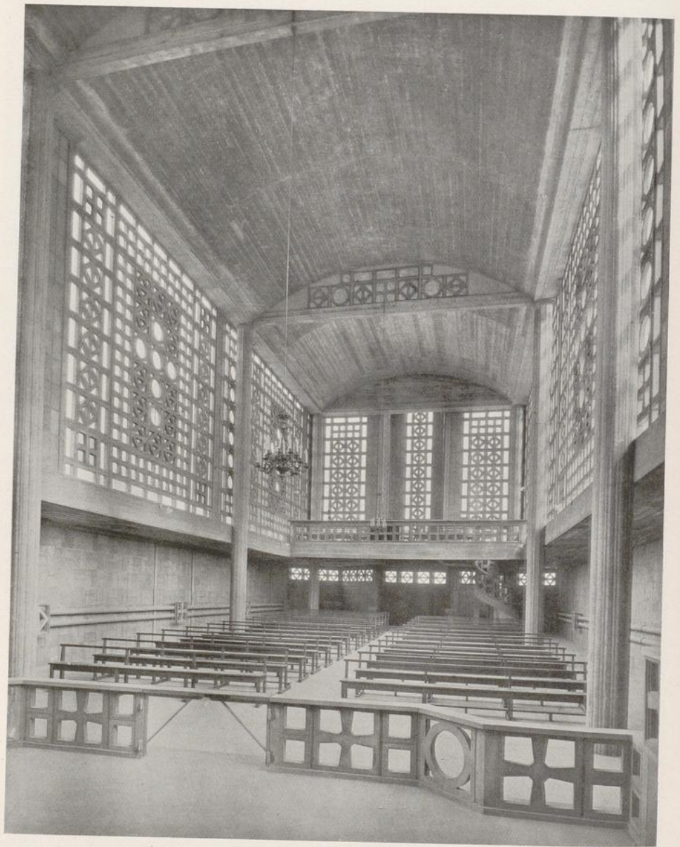
Auguste und Gustave Perret: Kirche Sainte-Thérèse, Montmagny bei Paris. 1925. (Eisenbeton)
