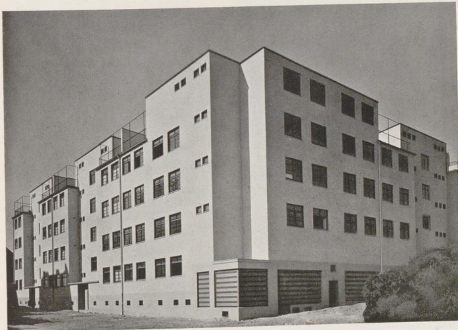
Wilhelm Riphahn und Caspar Maria Grod: Mehrfamilienhäuser, Köln-Mülheim. 1928
