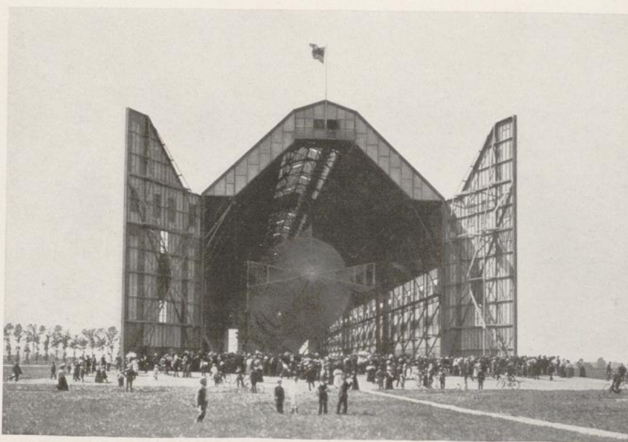
Luftschiffhalle, Baden-Oos. 1915. (Jetzt abgebrochen)
