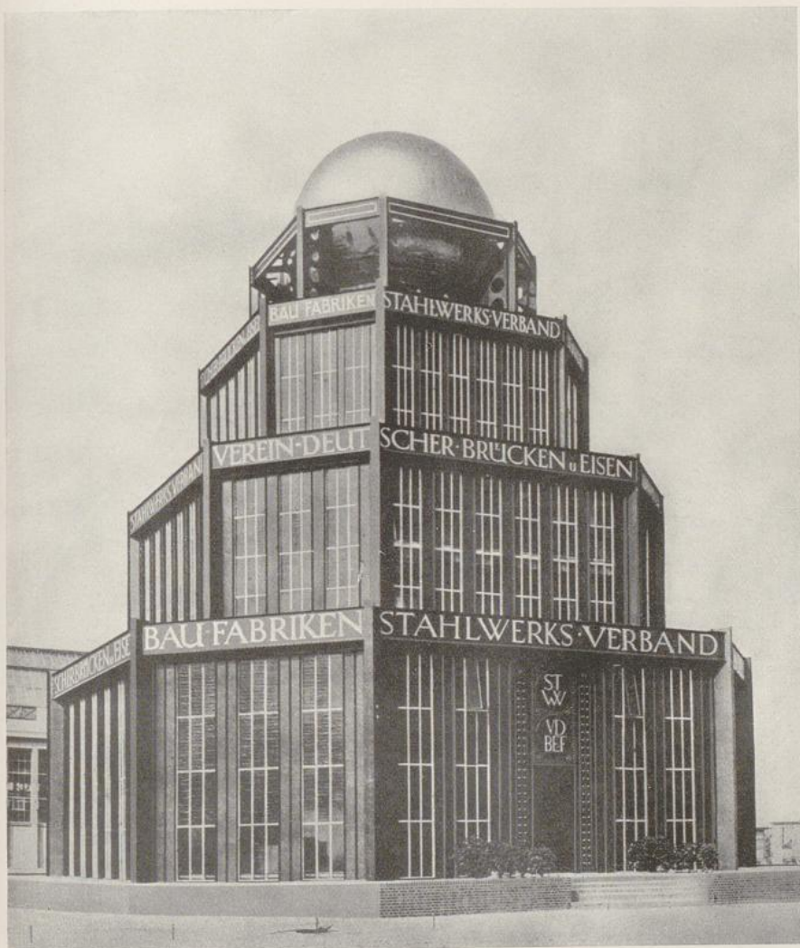
Bruno Taut und Franz Hoffmann: „Monument des Eisens“ Ausstellungspavillon auf der Baufach-Ausstellung, Leipzig, 1913
