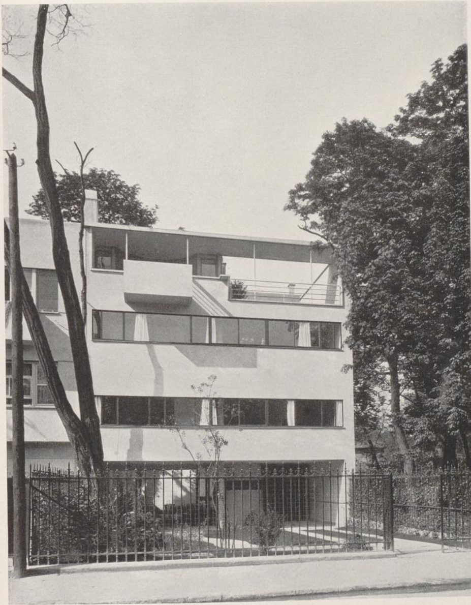
Le Corbusier und Pierre Jeanneret: Haus Cook, Boulogne-sur-Seine. 1926
