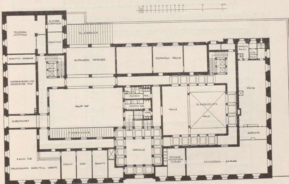
Grundriß des Erdgeschosses
