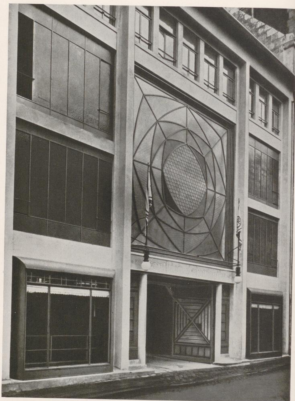
Auguste und Gustave Perret: Garage, Paris, Rue de Ponthieu. 1905. (Eisenbeton)
