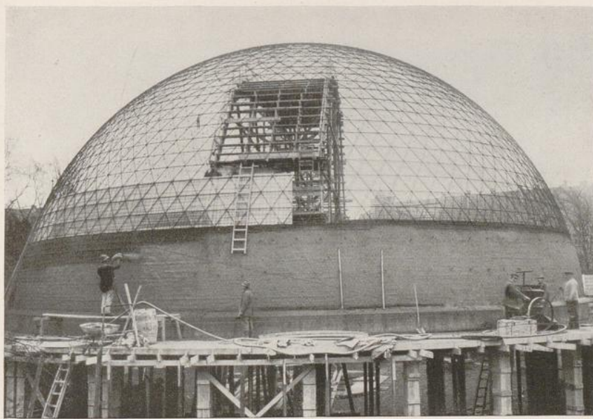
Fa. Dyckerhoff & Widmann: Planetarium, Jena. 1925. Konstruktion der Kuppel
