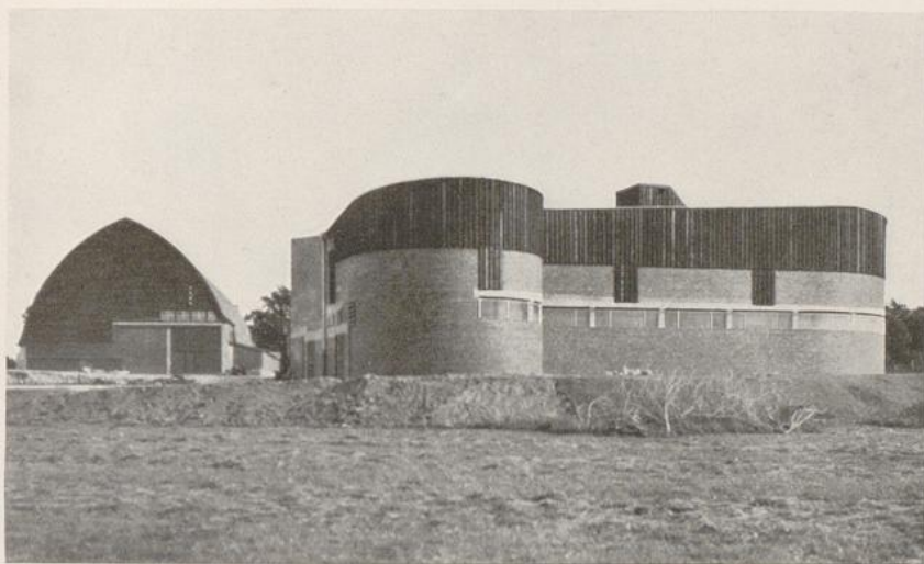
Hugo Häring: Viehhaus und Scheune, Gut Garkau. 1925
