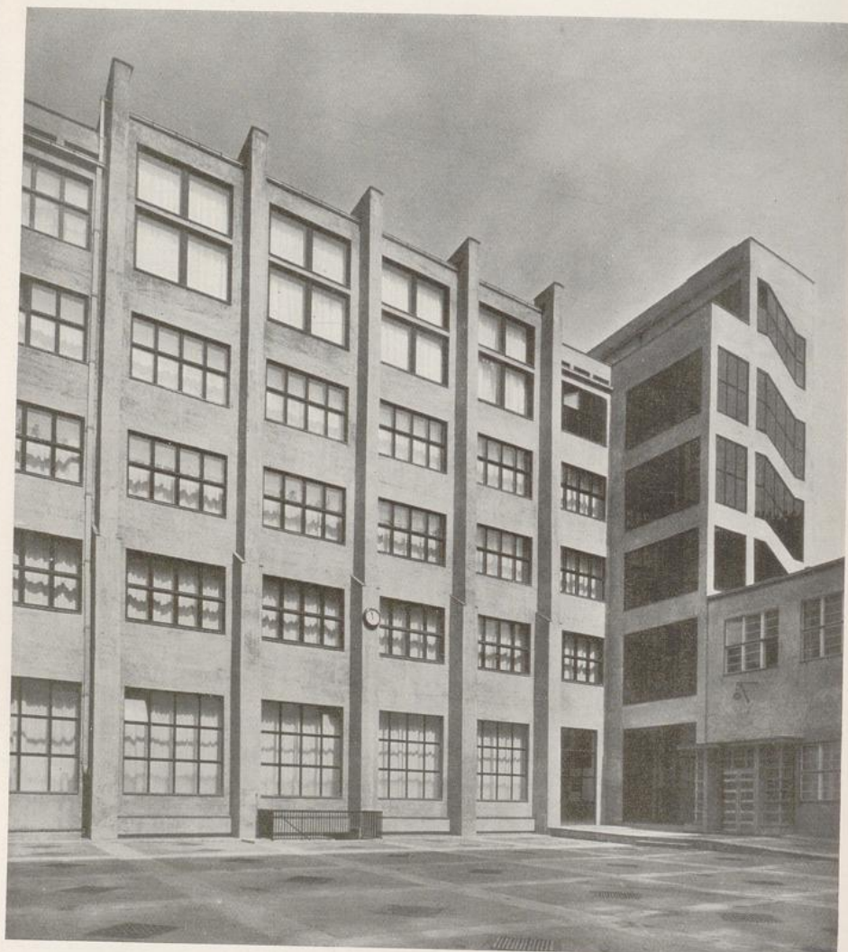
Max Taut: Verbandshaus der Deutschen Buchdrucker, Berlin. 1925. Hofansicht
