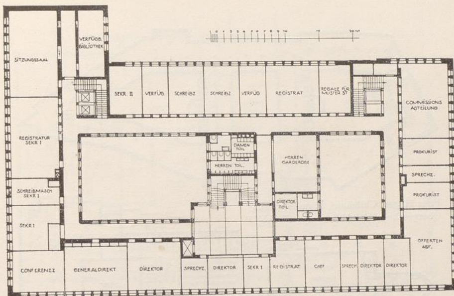
Grundriß des zweiten Obergeschosses
