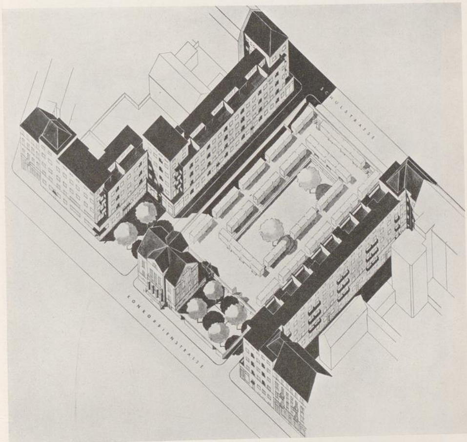
Gustav Adolf Platz: Plan für die Bebauung des Lamey-Geländes in Mannheim, unter Erhaltung des Lamey-Hauses. 1928
