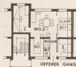
Gangwohnung der Siedlung Praunheim von Ernst May
