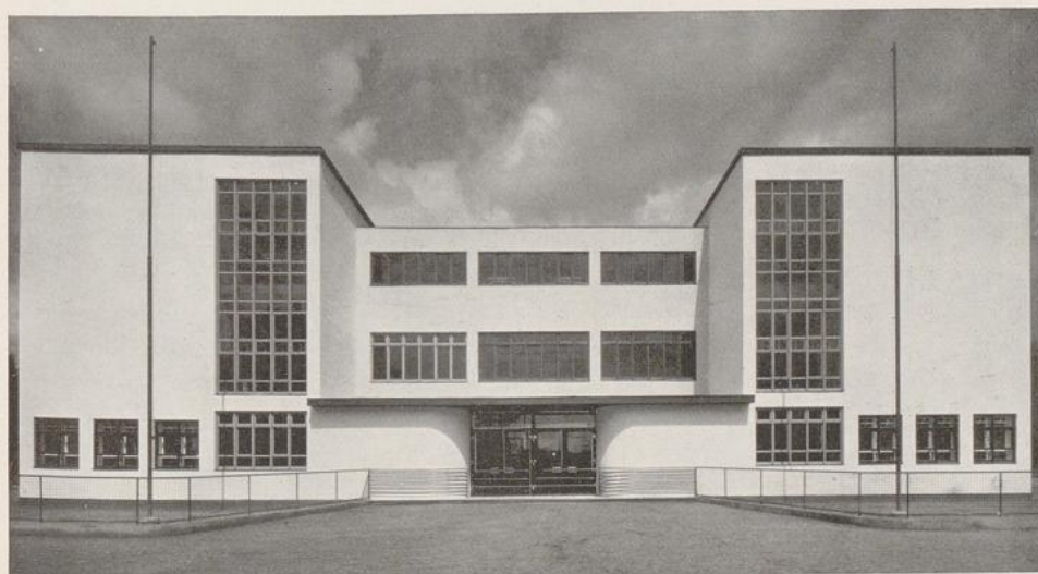
Otto Haesler: Volksschule, Celle. 1928. Hof- und Frontalansicht (Vgl. Grundrisse, Abb.586)
