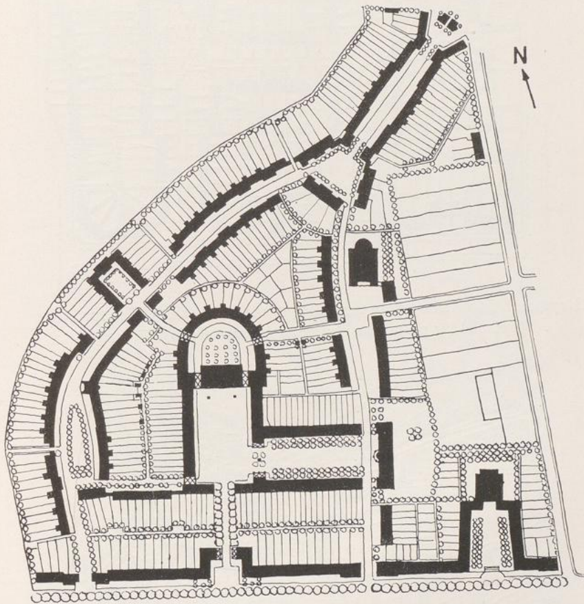
Otto Rudolf Salvisberg: Siedlung der Reichs-Stickstoff-Werke, Piesteritz bei Wittenberg. 1916. (Vgl. Abb. 340)
