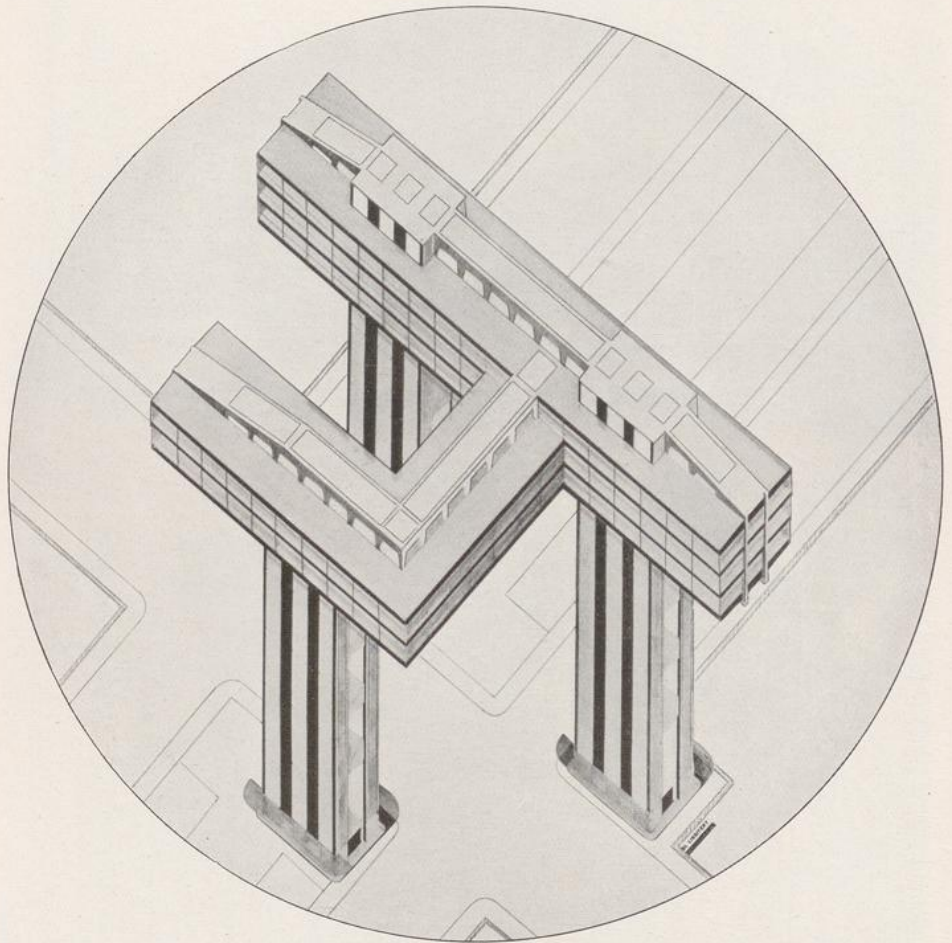
El Lissitzky: Hochhausentwurf „Wolkenbügel“. 1923
