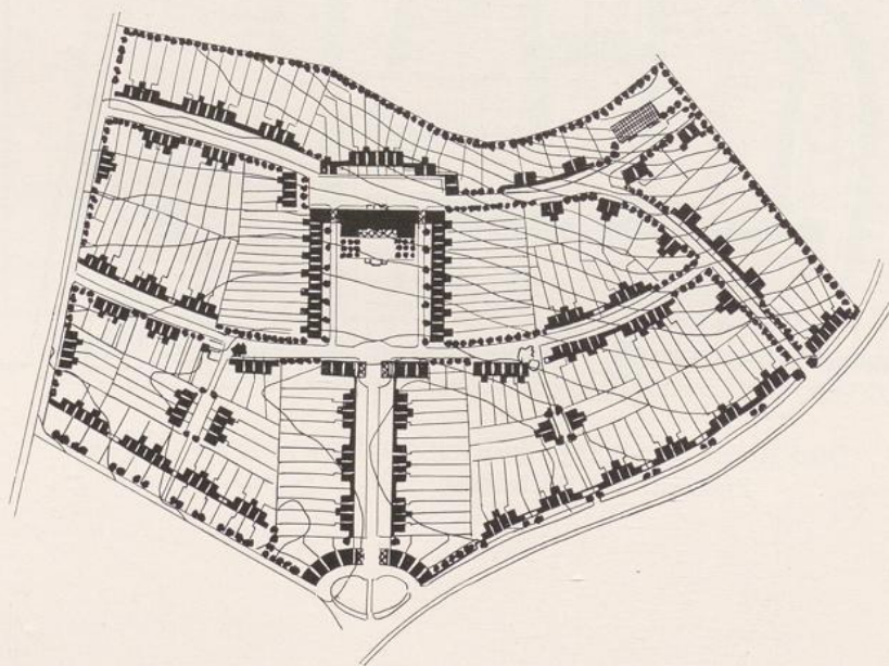
Otto Rudolf Salvisberg: Bebauungsplan für eine Arbeitersiedlung der Weinmann-Werke, Schwaz (Böhmen). 1921. (Vgl. Abb. 341)
