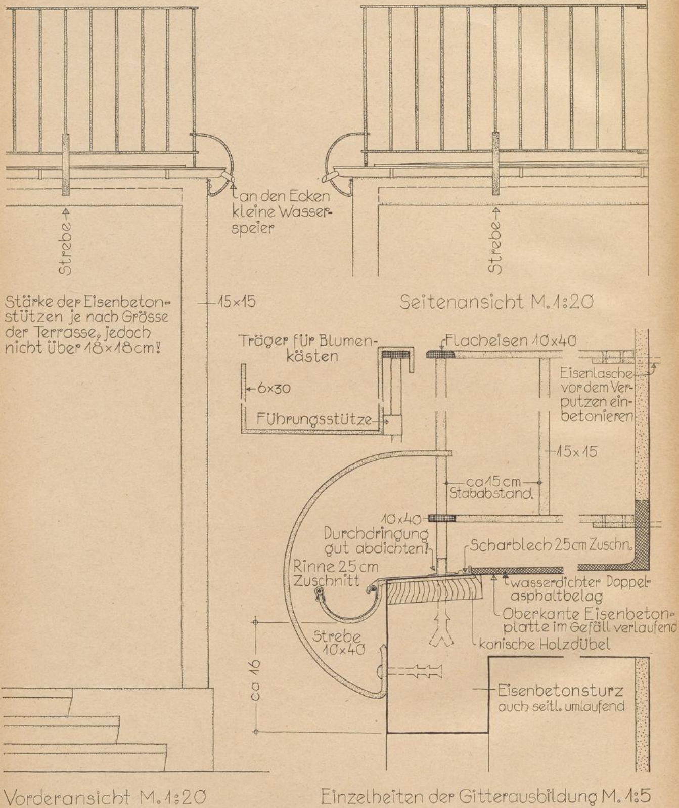
Tafel 18: Terrasse mit Eisengeländer M. 1:20 und 1:5
