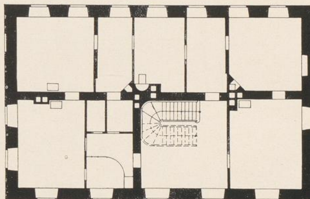
Erstes Obergeschoß
