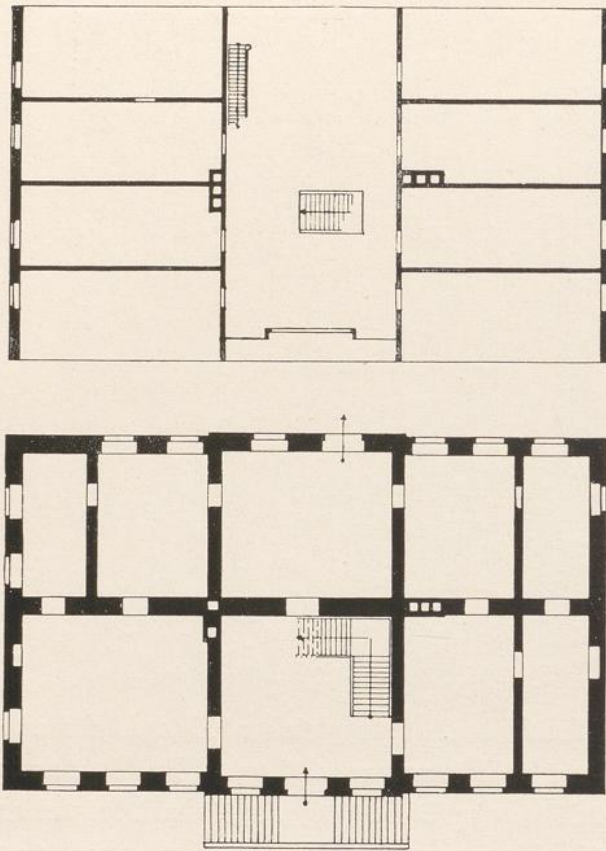
Abb. 15. Frauendorf. Obergeschoß u. Erdgeschoß Auf die Weise wurde der hintere Teil der Wohnraum, eine Art Gartensaal, frei.
