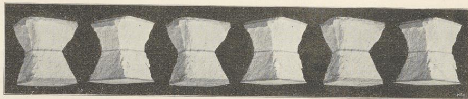
Druckversuch.
