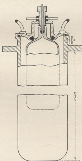
Fig. 249. Prüfung von Gasflaschen auf inneren Druck. Martens.
