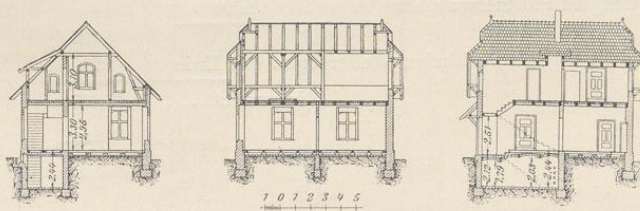
Fig. 40. Schnitte durch das Pförtnerwohnhaus.
