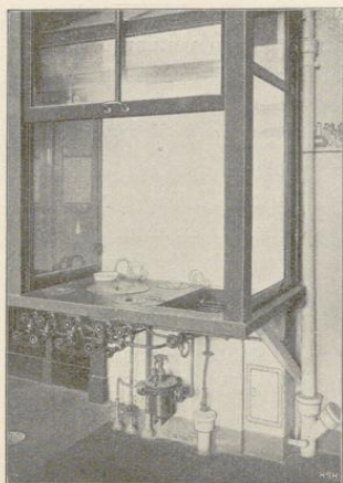
Fig. 166. Blick in und unter die Dampfkappe im Laboratorium der Abteilung für Ölprüfung.
