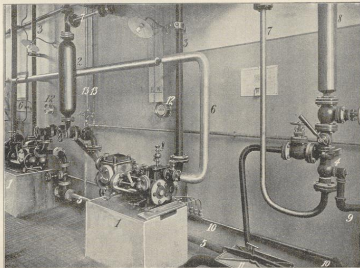
Fig. 144. Dampfpumpen und Injektor an der Ostwand des Kesselhauses.
