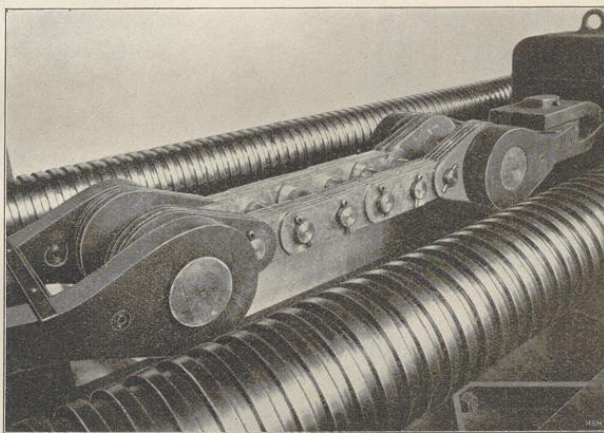
Fig. 245. Zugversuch mit einer Gallschen Kette.
