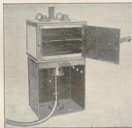
Fig. 140. Heißluftschränkchen in der Abteilung für Ölprüfung.
