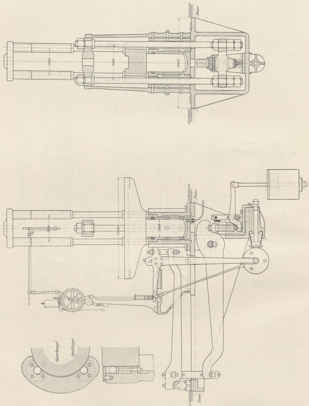
Fig. 261. Festigkeitsmaschine für 50000 kg Leistung von Pohlmeier. Heinr. Ehrhard-Düsseldorf.
