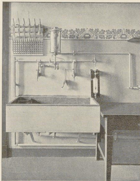
Fig. 115*). Holzbohtich mit Gasschnellwärmer* im chemischen Laboratorium der Abteilung für Ölprüfung (Raum 236).
