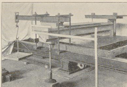
Treppenstufe, Drehversuch.
