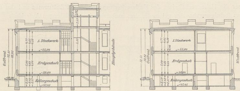
Fig. 29. Querschnitte durch das östliche Laboriengebäude.
