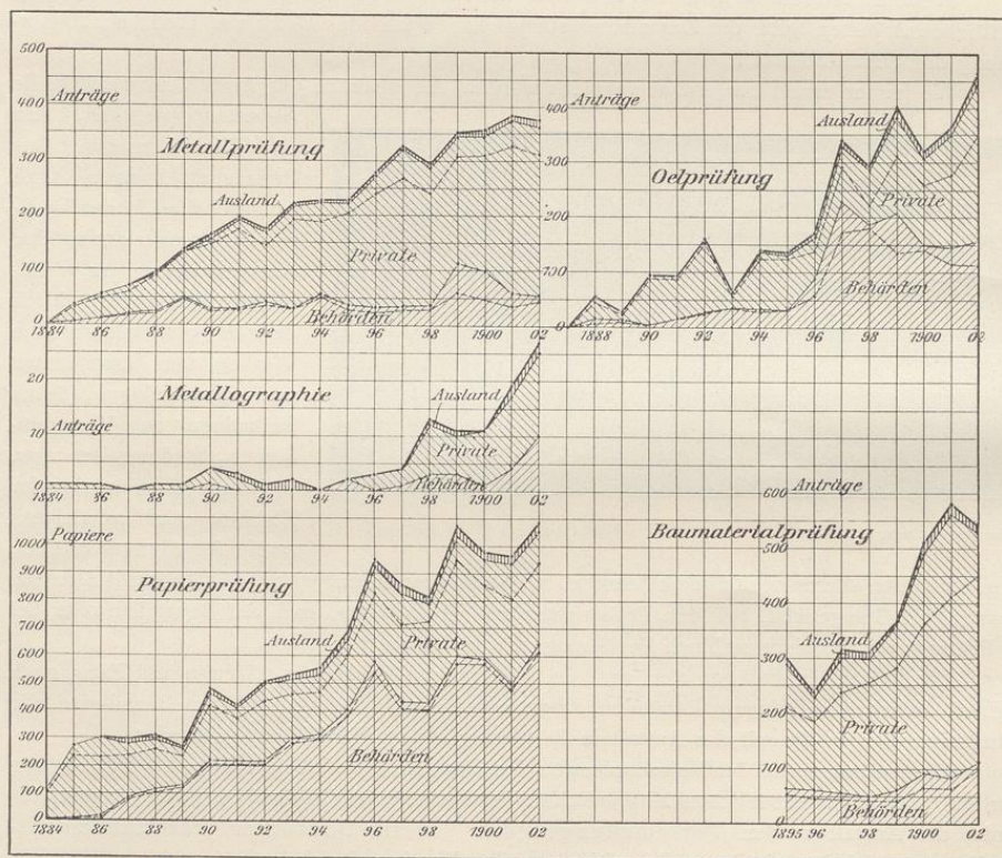
Fig. 4. Entwicklungsgang der Abteilungen in der Mechanisch-Technischen Versuchsanstalt. Die punktierten Linien innerhalb der Felder beziehen sich auf Preußen allein.
