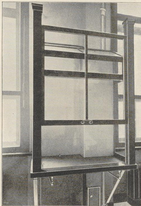
Fig. 91. Einteilige Wandkapelle am Fensterpfeiler des physikalischen Laboratoriums der Abteilung für Baumaterialprüfung (Raum 26).
