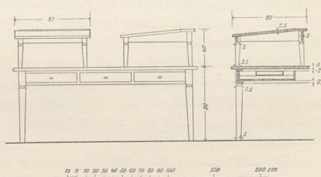
Fig. 105. Beweglicher Arbeitstisch mit abnehmbarem Schreibpult.
