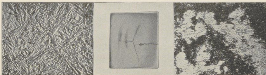
Überhitzt gehärteter Werkzeugstahl.
