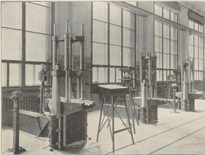
Fig. 256. 100000 und 50000 kg Probiemaschinen von Pohlmeier. Heinr. Ehrhardt-Düsseldorf.
