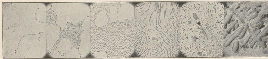
0,08 1,16 1,78 3,5 4,7 9 0/0 Cu 2 O Kupfer- und Sauerstoff.
