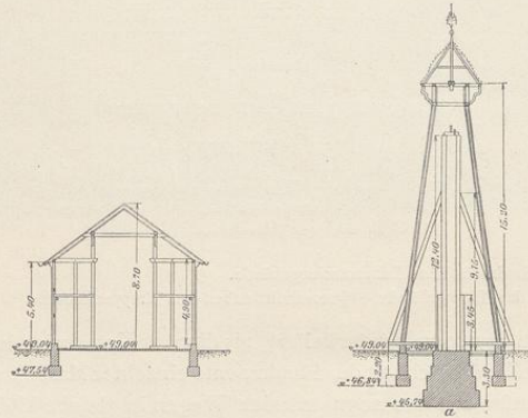
Fig. 34. Querschnitt durch den Fallwerkschuppen mit Fallwerkurm. (a Fundament der Chabotte des großen Fallwerks.)
