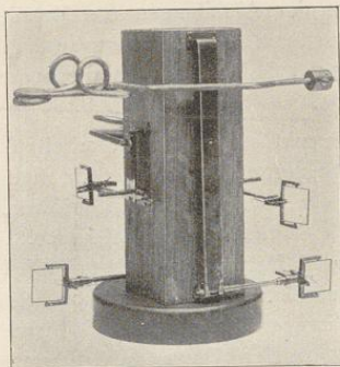
Elastizitätsbestimmung.
