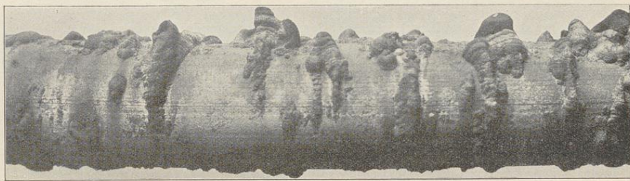
Rost auf Wasserschlange
