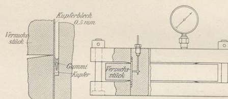
Fig. 252. Prüfung dicker Ringe auf inneren Druck. Martens.
