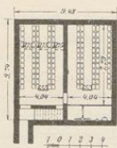
Fig. 174. Akkumulatorenräume (652 und 653) und Raum für den Zellschalter. (654 u. 655). [Vgl. Fig. 14.]
