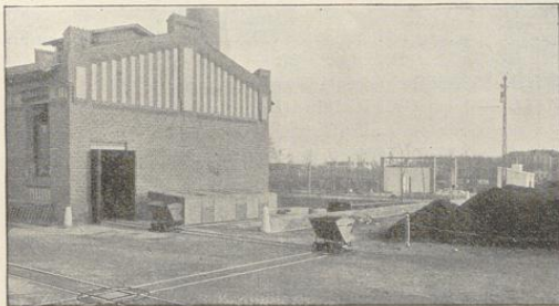
Fig. 193. Gleisanlagen vor dem Kohlenhof und Kesselhaus.
