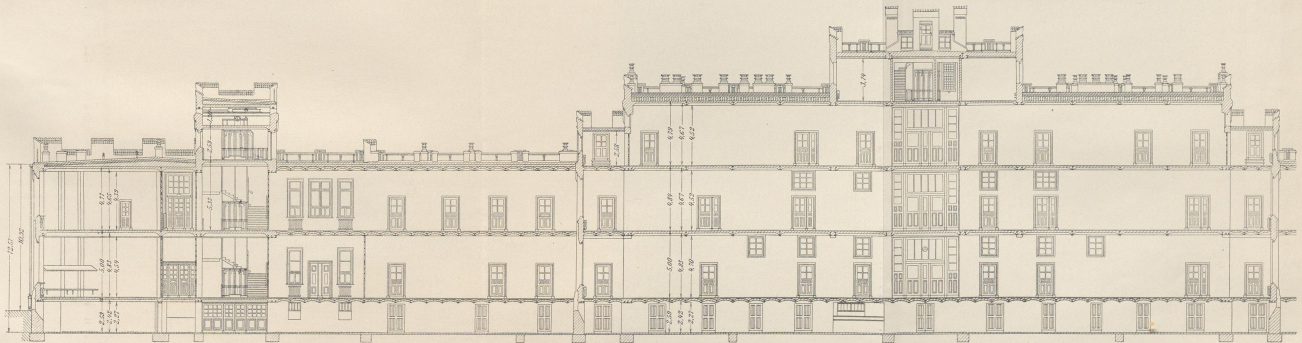
Schnitt durch das östliche Laboratoriengebäude und durch das Hauptgebäude (nach Süden gesehen).
