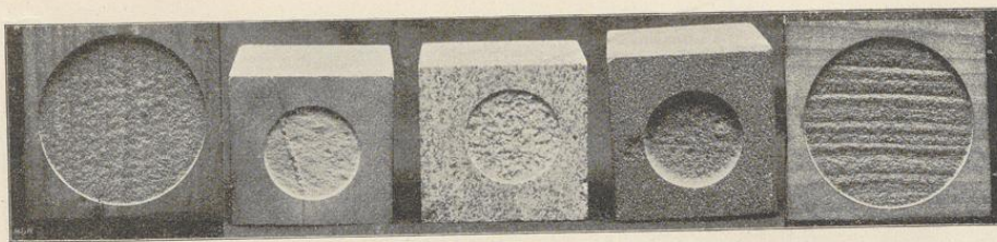
Abnutzung durch Sandstrahl.
