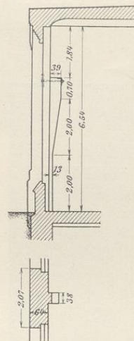
Fig. 57. Unterstützungspfeiler für die Laufräger der Krane.
