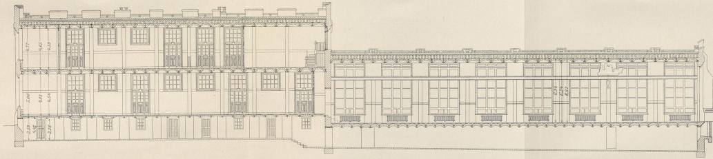
Längsschnitt durch das östliche Laboratoriengebäude und die östliche Versuchsstätte (nach Osten gesehen).
