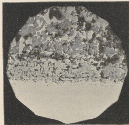
Schwefeleisenbildung auf Siederohr.
