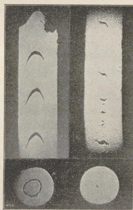
Unganzer Draht.
