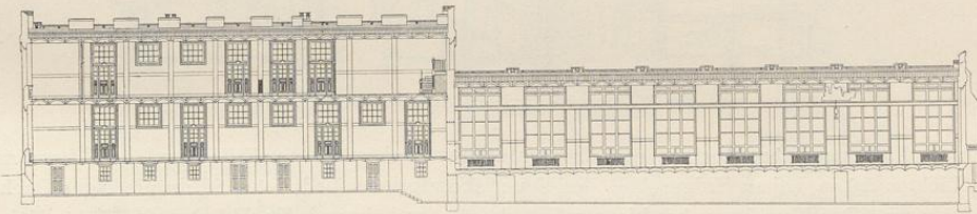
Fig. 30. Längenschnitt durch das Laboriengebäude und die Versuchsstätte.
