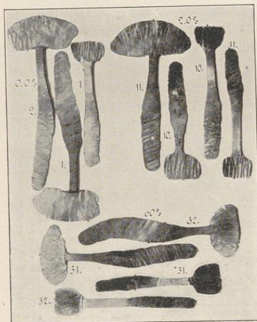
Ausbreitproben, Hufnägel.
