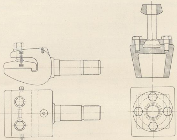
Fig. 267. Einspannung für Riemen von Martens. Maschinenbaugesellschaft Nürnberg.
