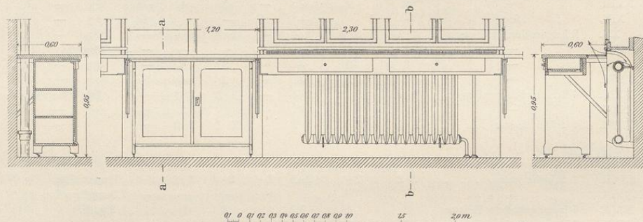
Fig. 98. Fensterarbeits-tische und Fensterpfeilerschränkchen.
