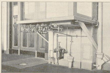
Fig. 166. Blick in und unter die Dampfkappe im Laboratorium der Abteilung für Ölprüfung.
