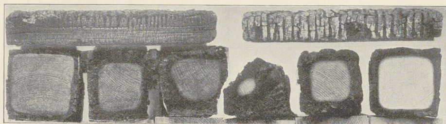
Brandversuche.
