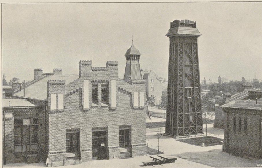
Fig. 45. Maschinenhaus und Kühlturm von Nordwesten aus gesehen.
