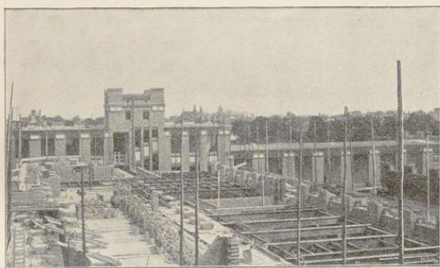
Fig. 58. Verlegen der Träger im Hauptgebäude und in der westlichen Versuchsstätte.
