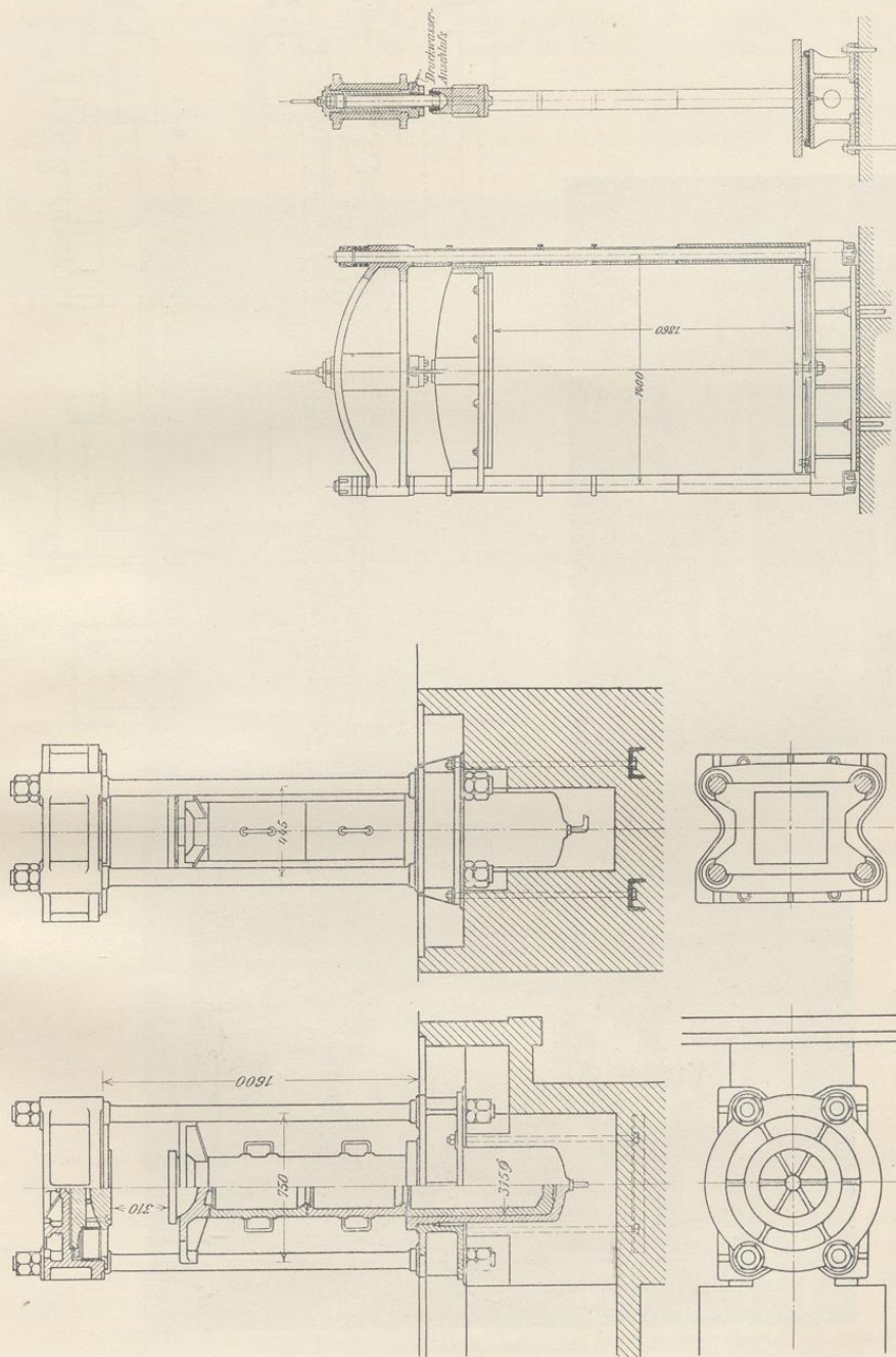
Fig. 319. 20 000 kg-Rohrprüfmaschine von Martens. A. Borsig-Tegel.
