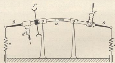
Fig. 294. Dauerversuche mit erhitzten Kupferrohren von Rudeloff.
