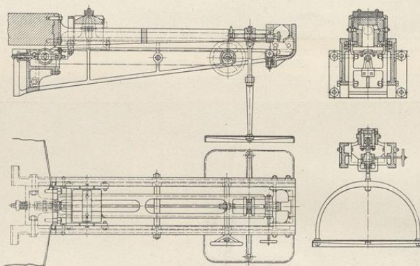
Fig. 259. Laufgewichtswage zur Werdermaschine.
