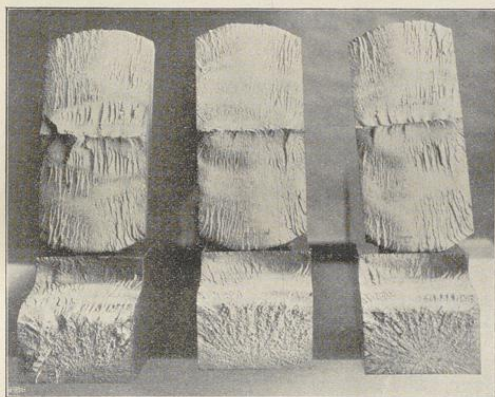
Biegeversuch.
