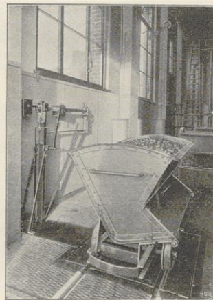
Fig. 195. Zentesimalwaage im Kesselhause.
