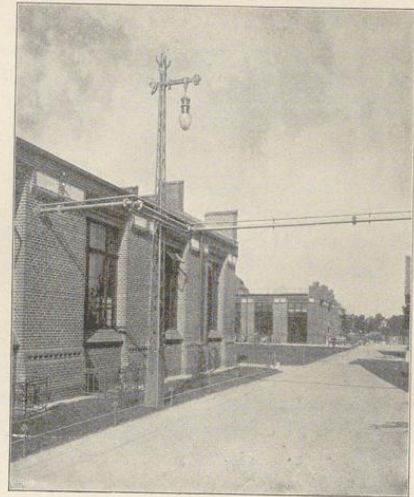
Fig. 152. Maschinenhaus mit der Warmwasserleitung und der Abdampfleitung von den Pumpen nach dem Kühlturm.
