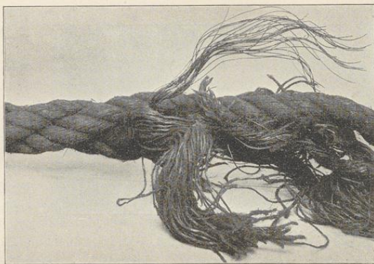
Zerreißversuch, Hanfseil.
