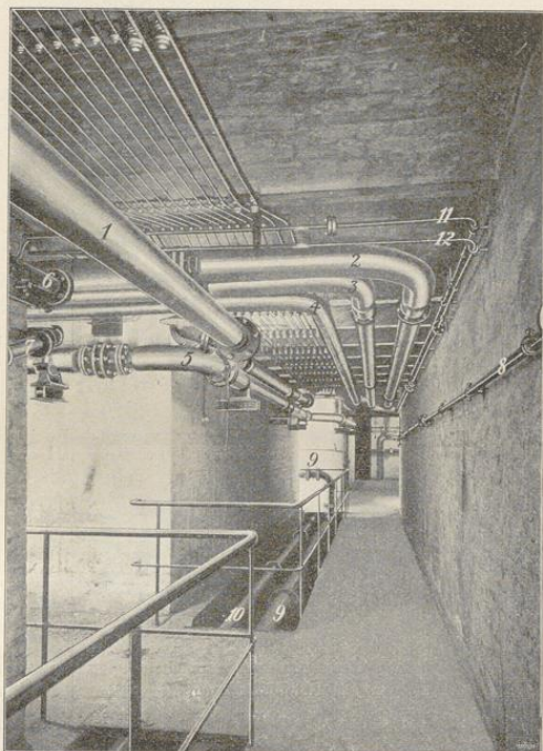
Fig. 153*). Röhrenkeller zwischen dem Sammelbassin unter dem Kühlturm und dem Reinigungsbassin neben demselben.
