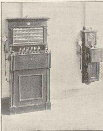
Fig. 188. Umschalterschrank für die Hausanschlüsse und Umschalterschrank für die Postanschlüsse der Fernsprechanlage. (No. 6 und 7 der Figur 185.)
