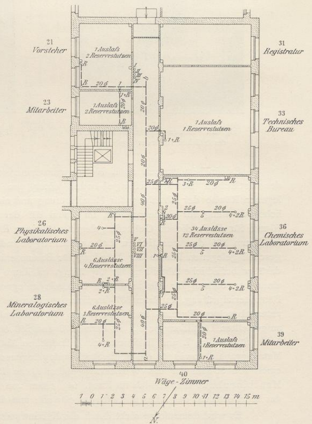
Fig. 128. Betriebswasserleitung im Erdgeschoß des westlichen Laboratoriengebäudes mit den Entnahmestellen in diesem Geschoß.
