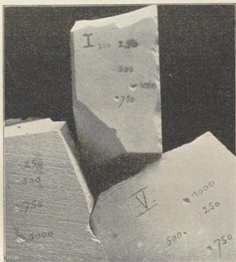
Härteprüfung, Porzellanwalzen.
