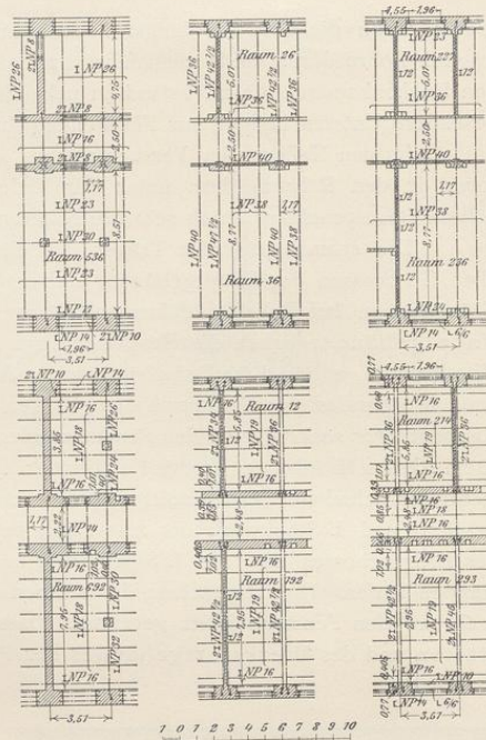
Fig. 61. Lage der Träger in den Laboriengebäuden und im Hauptgebäude.
