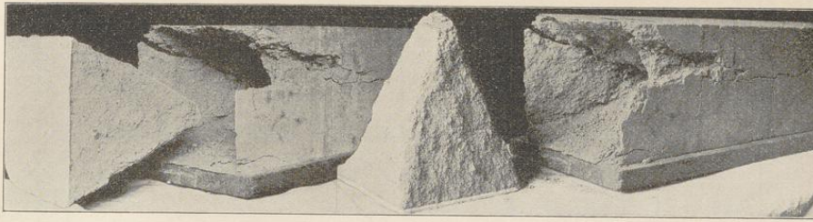
Druckversuch mit Betonsäule.
