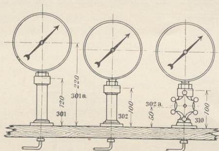
Fig. 206. Manometer-Aufstellung.
