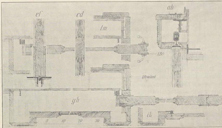
Fig. 86. Einzelheiten der Schiebetüren. (Vgl. Figur 87.)
