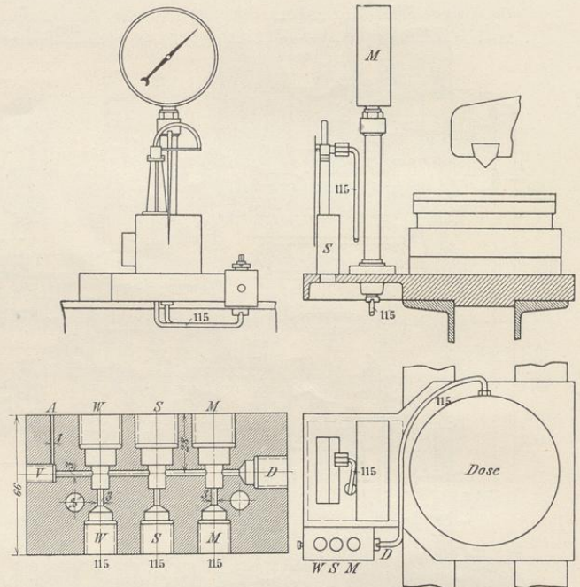
Fig. 214. Steuerung zur Drehfestigkeitsmaschine von Martens.
