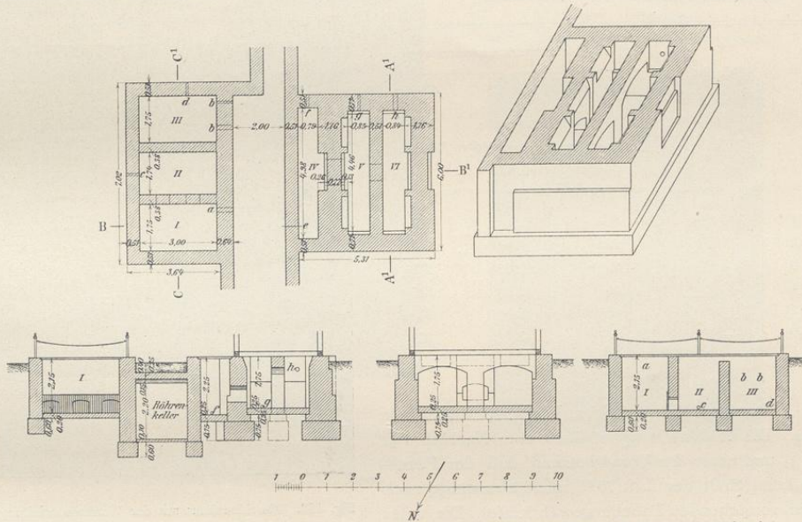
Fig. 151. Reinigungsbassin neben dem Kühlturm und Sammelbassin unter demselben (I, II, III Reinigungsbassin — IV, V u. VI Sammelbassin).
