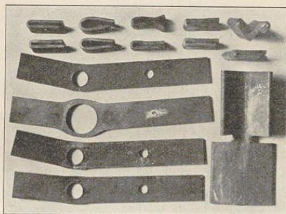
Technologische Proben.
