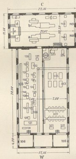
Fig. 287. Werkstatteingebäude CW.
