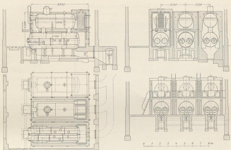
Fig. 141. Grundrisse und Schnitte der Dampfkesselanlage im Kesselhause.
