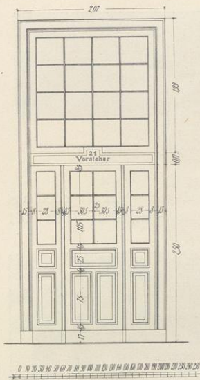
Fig. 89. Dreiteilige Flurtüren mit Oberlicht in den Laboratoriengebäuden.
