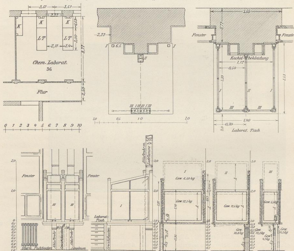
Fig. 94. Fensterfeilerdoppelkapellen.
