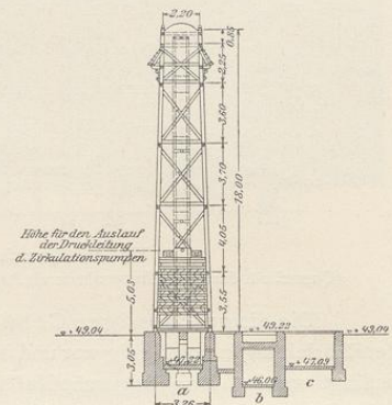
Fig. 35. Querschnitt durch den Kühlturm mit dem Sammelbassin a, durch den Röhrenkeller b und durch das Reinigungsbassin c.
