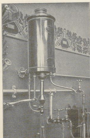
Fig. 139. Gasschnellwärmer, System Prof. Junkers.
