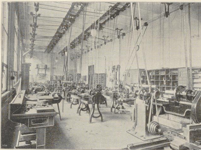
Fig. 296. Mechanische Werkstatt W 103 Innenansicht.
