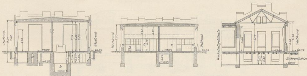
Fig. 31. Schnitt durch die östliche Versuchsstätte (a Fundament der 500 t-Maschine [Hoppe] b Fundament der Rohrprüfungsmaschine [Borsig]).
