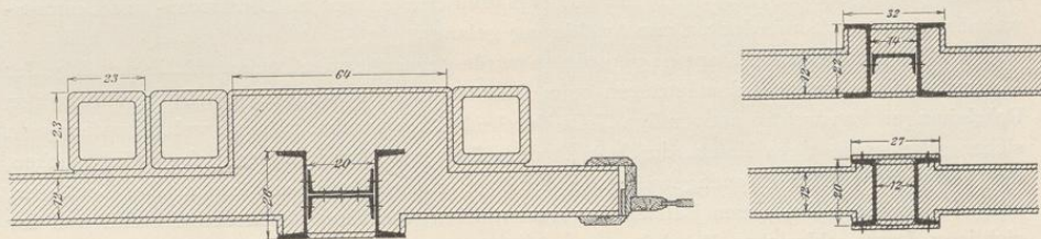
Fig. 56. Schnitte durch die eisernen Stützen in den Laboriengebäuden, in den Versuchsstätten und im Werkstattgebäude.
