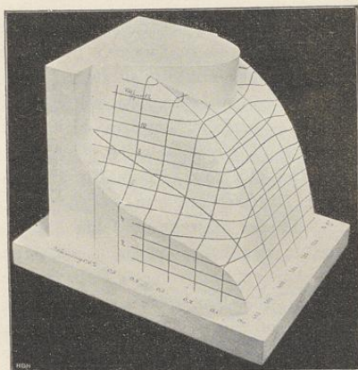
Festigkeit erhitzten Eisens.
