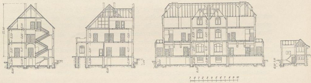
Fig. 38. Schnitte durch das Direktorenwohnhaus.
