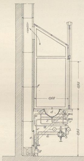
Fig. 166. Blick in und unter die Dampfkappe im Laboratorium der Abteilung für Ölprüfung.
