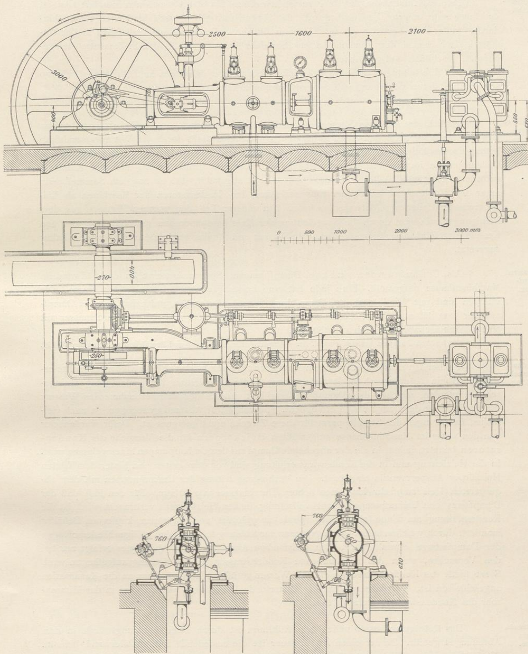
Fig. 150. Dampfmaschinen (Ansicht, Grundriß und Schnitte).
