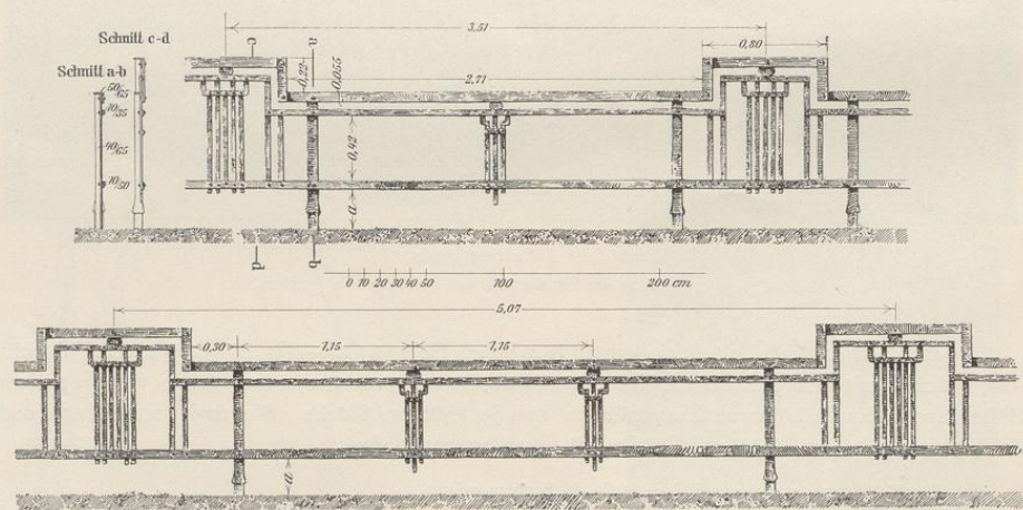
Fig. 67. Schmiedeeiserne Dachgitter auf den Laboriengebäuden, und dem Hauptgebäude sowie auf den Versuchsstätten.
