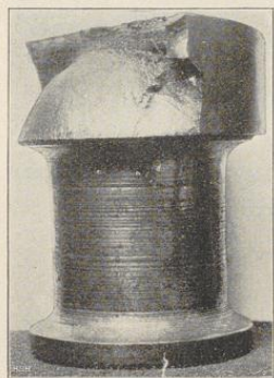
Krummzapfenbruch.
