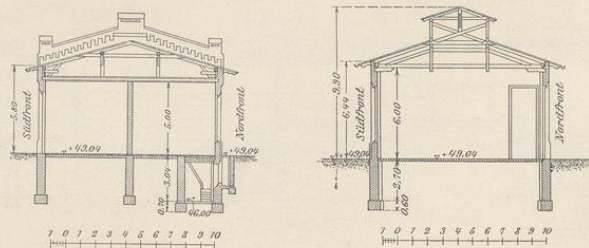
Fig. 37. Querschnitte durch das Feuerlaboratorium und das Kesselhaus.
