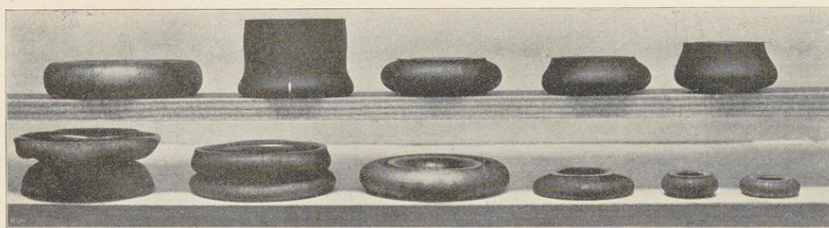
Stauchversuch, gezogene Röhren.
