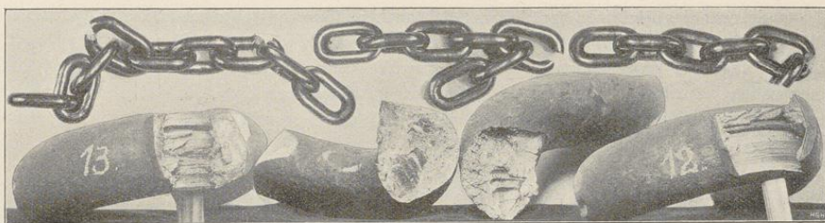
Kettenprüfung.
