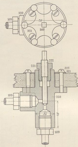
Fig. 233. Absperrventile.
