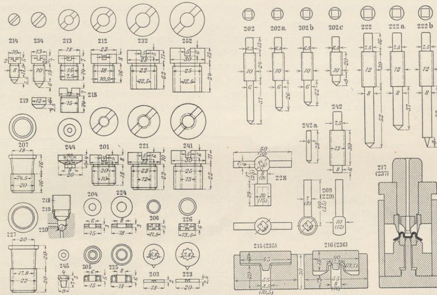
Fig. 209. Normalien für die Steuerungen.
