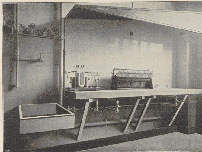
Fig. 103. Verbrennungstisch mit Gasometerbottich in der Abteilung für Ölprüfung (Raum 228).
