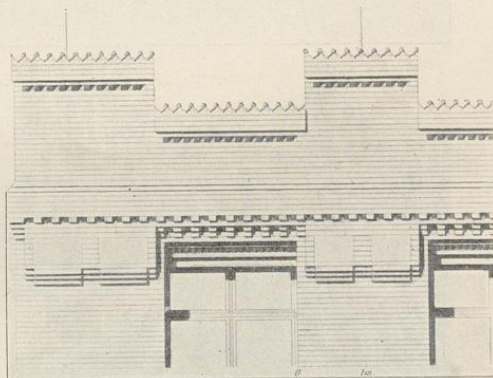
Fig. 44. Hauptgesims an den nördlichen Stirnseiten der Laboratoriengebäude.
