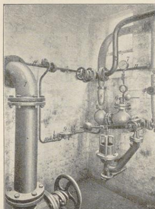
Fig. 155***). Röhrenkeller zwischen dem Reinigungsbassin und dem Sammelbassin.
