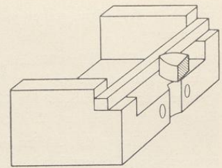
Fig. 286. Ambos für Schlagbiegeversuche mit dem Pendelhammer.
