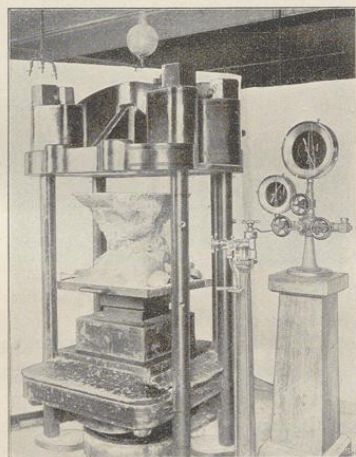
Alte Druckpresse.
