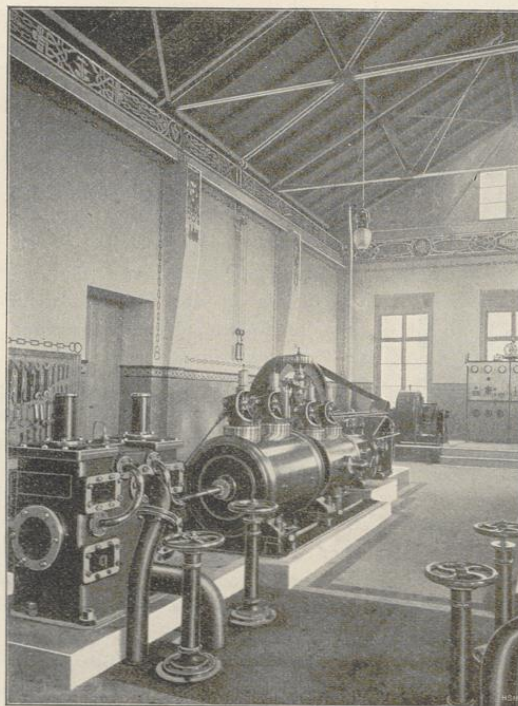
Fig. 149. Das Maschinenhaus mit der an der Nordseite desselben montierten Dampf- und Dynamomaschine.
