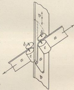
Fig. 338. Grundsatz des Schopperschen Falzers.
