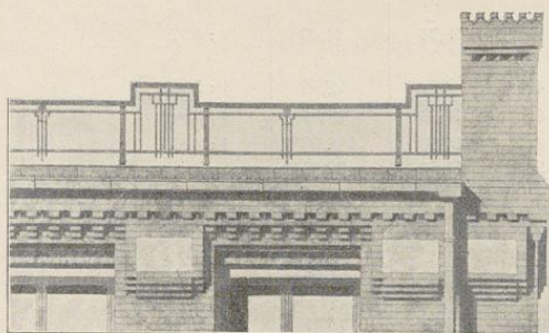
Fig. 42. Hauptgesims an der Längsfront des östlichen Laboratoriengebäudes.
