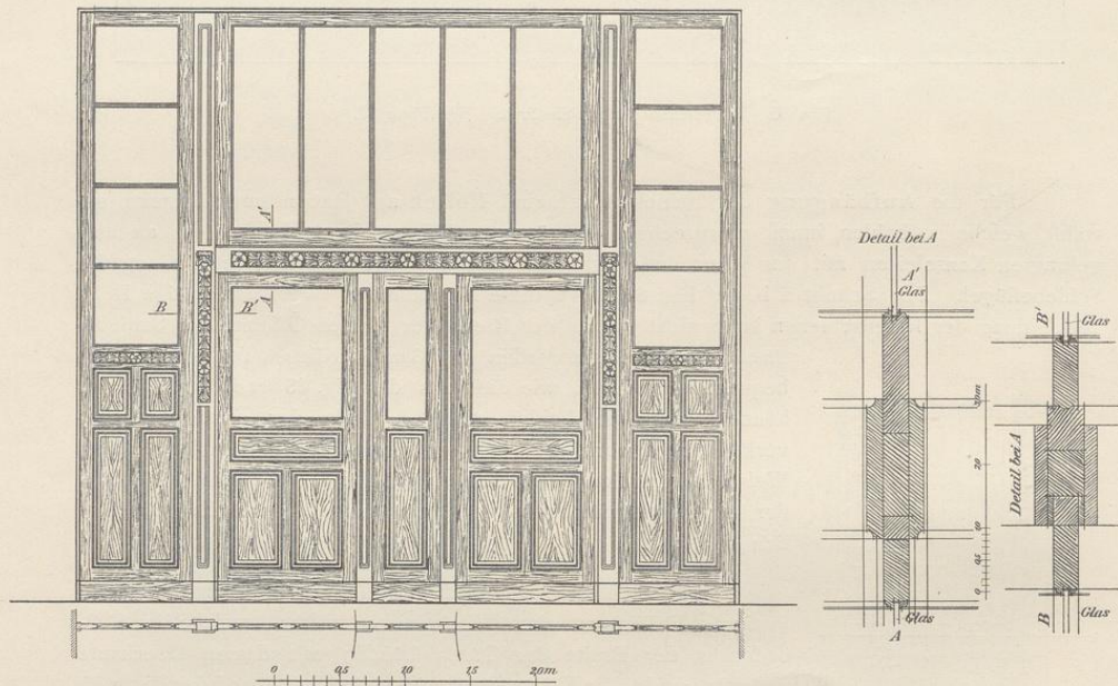
Fig. 88. Abschlußwand im Windfang des Hauptgebäudes mit zwei einflügeligen Pendeltüren und herausnehmbarem Zwischenteil (Vgl. Fig. 191 und 192 Seite 268).
