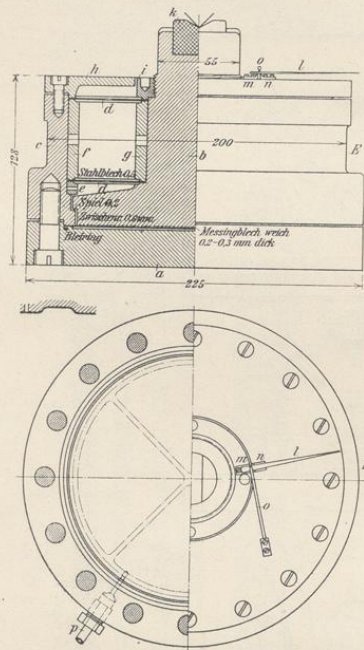
Fig. 213. Meßdose von Martens.
