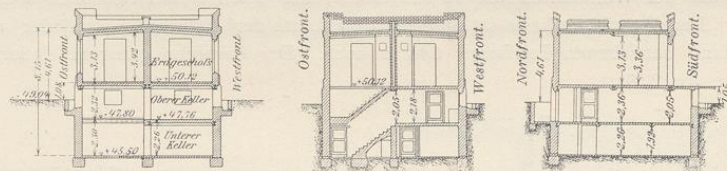
Fig. 36. Schnitte durch das Akkumulatorenhaus.
