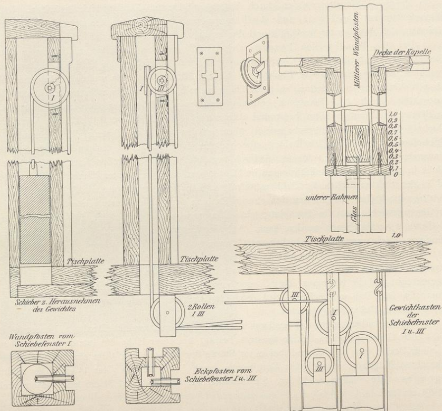
Fig. 95. Einzelheiten der Fensterfeilerdoppelkapellen.
