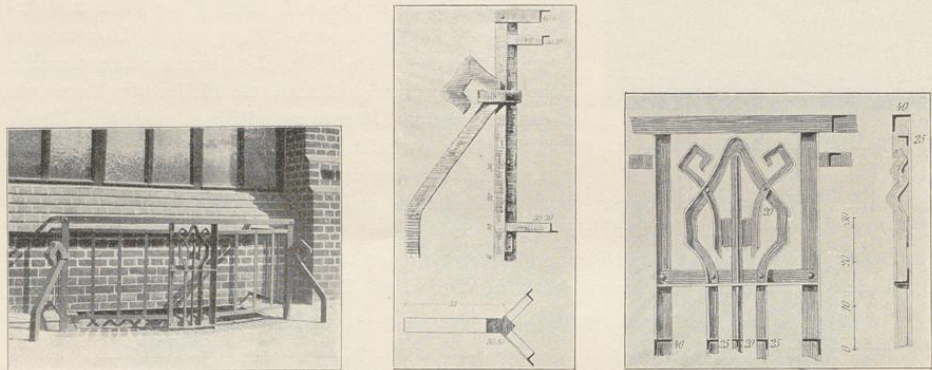
Fig. 201. Schmiedeeiserne Vergitterungen der Kellerlichtkränze.
