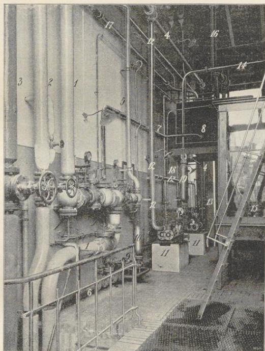
Fig. 148*). Pumpen und Leitungen an der Ostwand des Kesselhauses.
