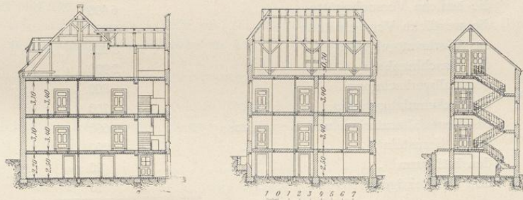
Fig. 39. Schnitte durch das Beamtenwohnhaus.
