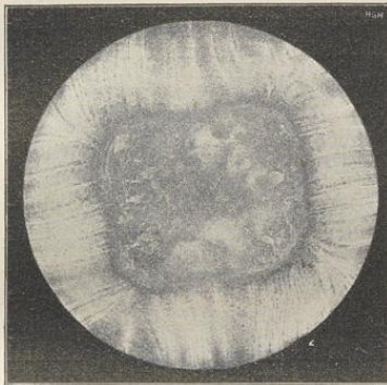
Zonenbildung in Flußeisen.
