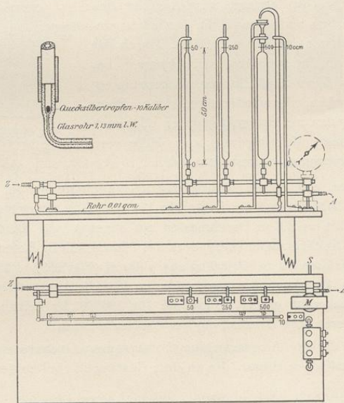
Fig. 250. Messung der Formänderung durch Wasserverdrängung nach Martens.
