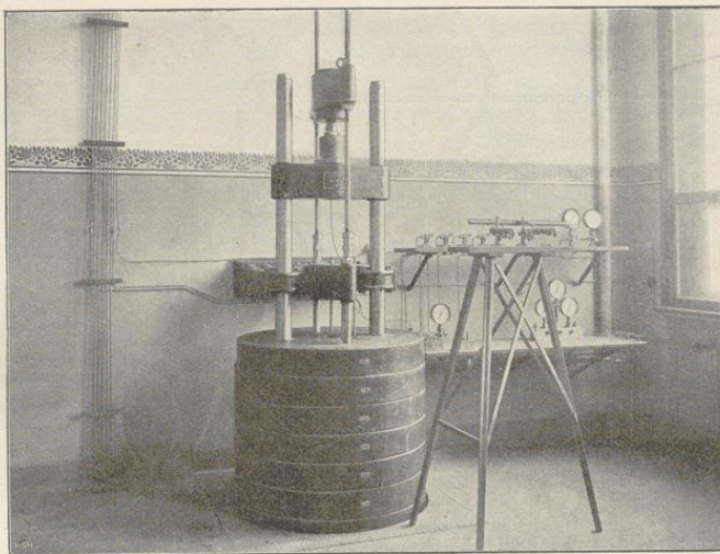
Fig. 248. Kontrollstab- und Manometerprüfung.
