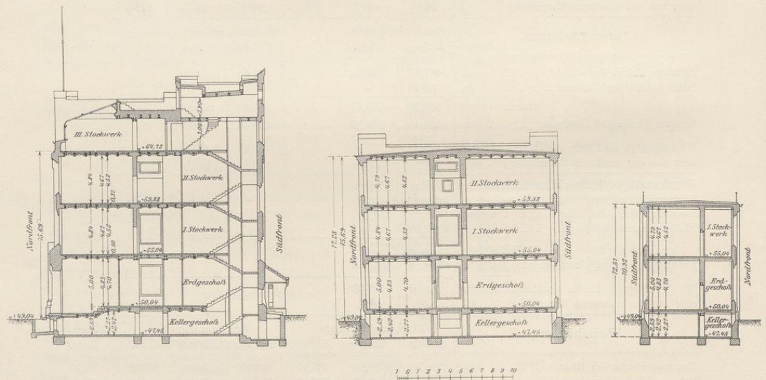
Fig. 28. Querschnitte durch das Hauptgebäude. (Mittelbau mit Atelier und Treppenhaus — Mittelbau neben dem Atelier — Flügelbau.)
