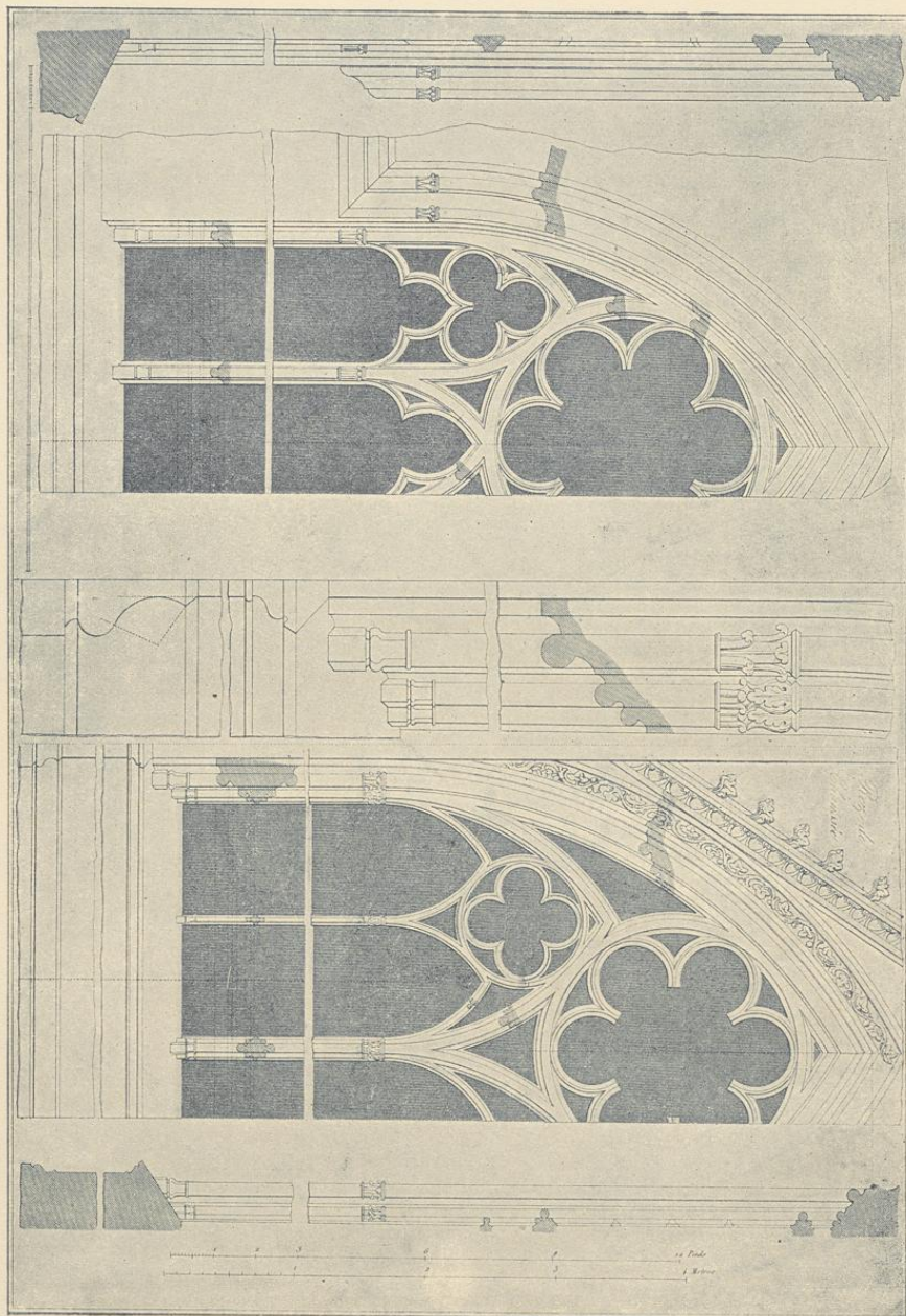
Fig. 257. Notre Dame Paris. Details des Masswerkes (Lassus und Viollet-le-Duc, Monogr. de N. D.).
