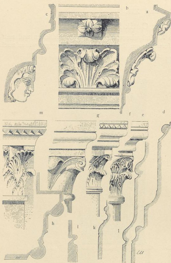
Fig. 248. Kathedrale zu Chartres. a b) Details der Rosette der nördlichen Fassade c d e g h i k l) Details des alten Glockenturmes m f) Kapitäl am neuen Glockenturm.
