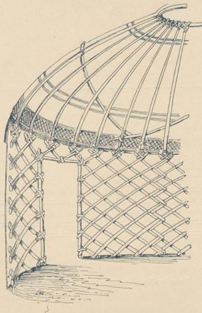
Fig. 122. Lattengerüst eines Kirgisentzel.
