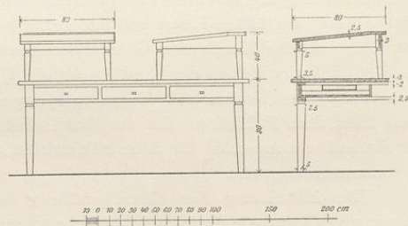
Fig. 105. Beweglicher Arbeitstisch mit abnehmbarem Schreibpult.
