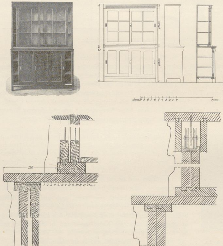
Fig. 109. Apparatschrank mit Schiebetüren.
