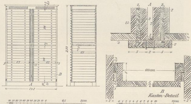
Fig. 112. Plattenschränk für Negative im photographischen Atelier.
