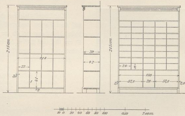
Fig. 113. Regale für Akten und Vordrucke.
