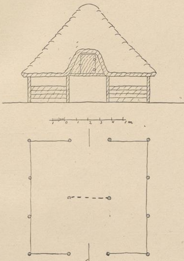
Abb. 9. Quadratische Form.
