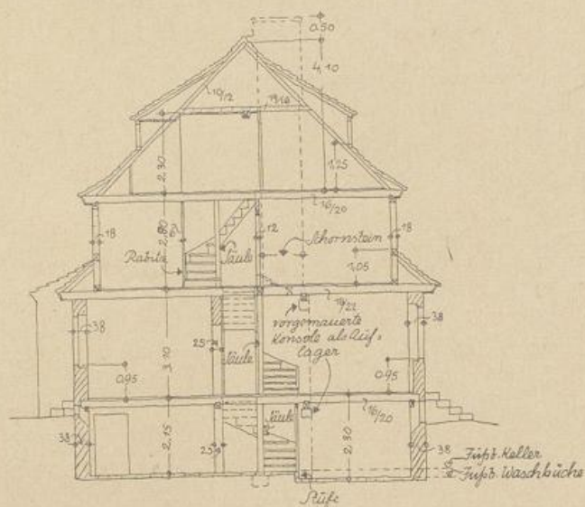
Querschnitt a-b
