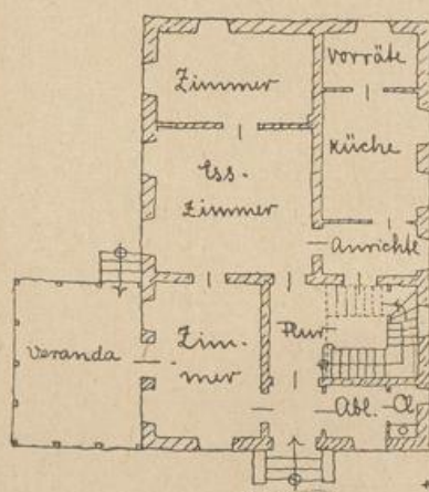
Beispiel 2: Erdgeschossgrundriß.
