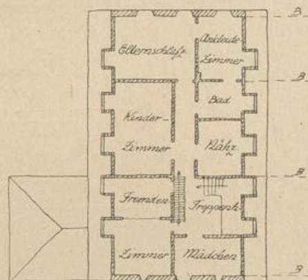
Beispiel 2: Dachgeschossgrundriß.
