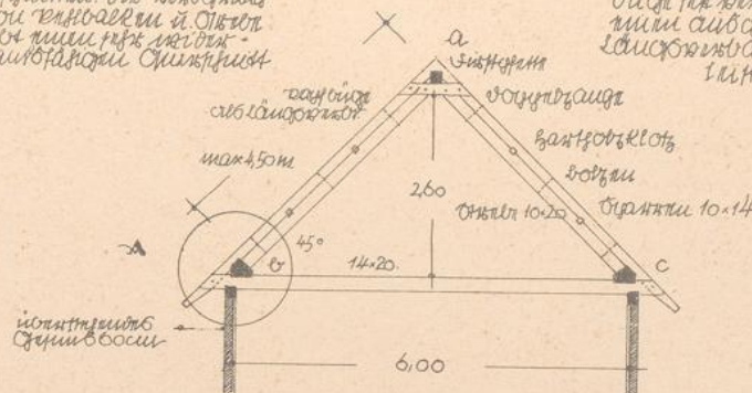
LIEGENDER DACHSTUHL * 1:100
