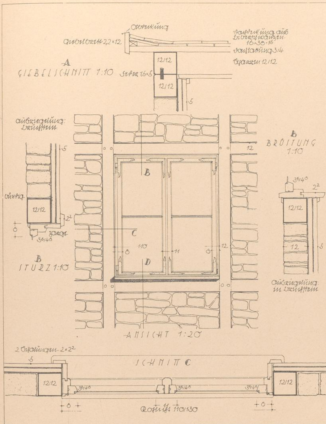
Das Fenster im zweigeschossigen Fachwerkhaus und ein Giebelschnitt
