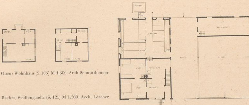
Wohnhaus (S. 107) M 1:300, Arch. Schmitthenner
