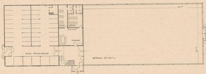
Reithalle (S. 131) M 1:500, Arch. Wetzel
