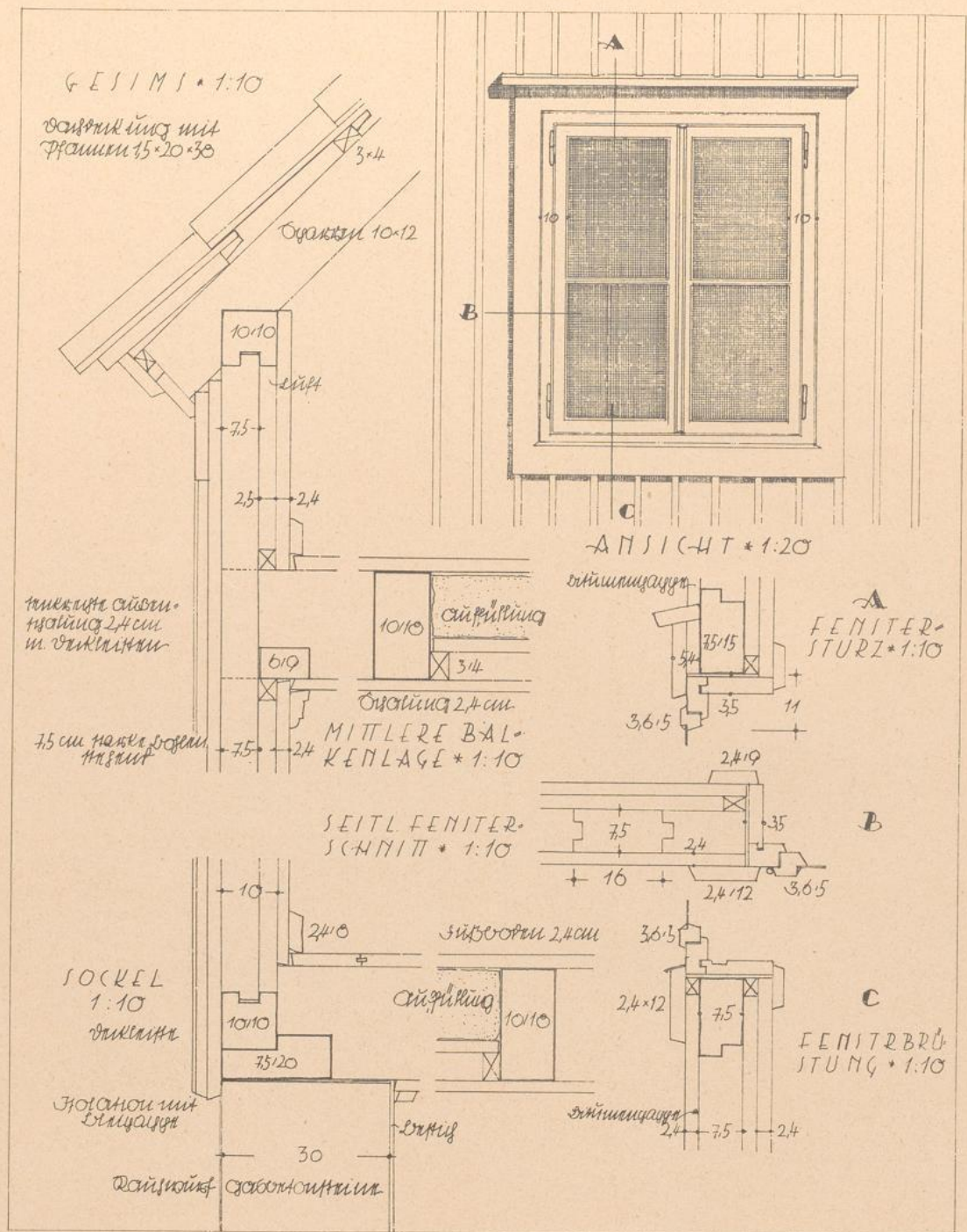
Zweigeschossiger schwedischer Bohlenbau: Fenster und wichtigste Schnitte
