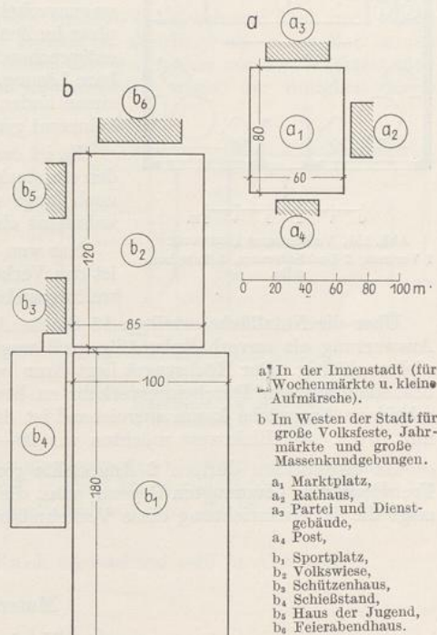
Abb. 150. Aufmarschplatz, Marktplatz (schematische Darstellung).
