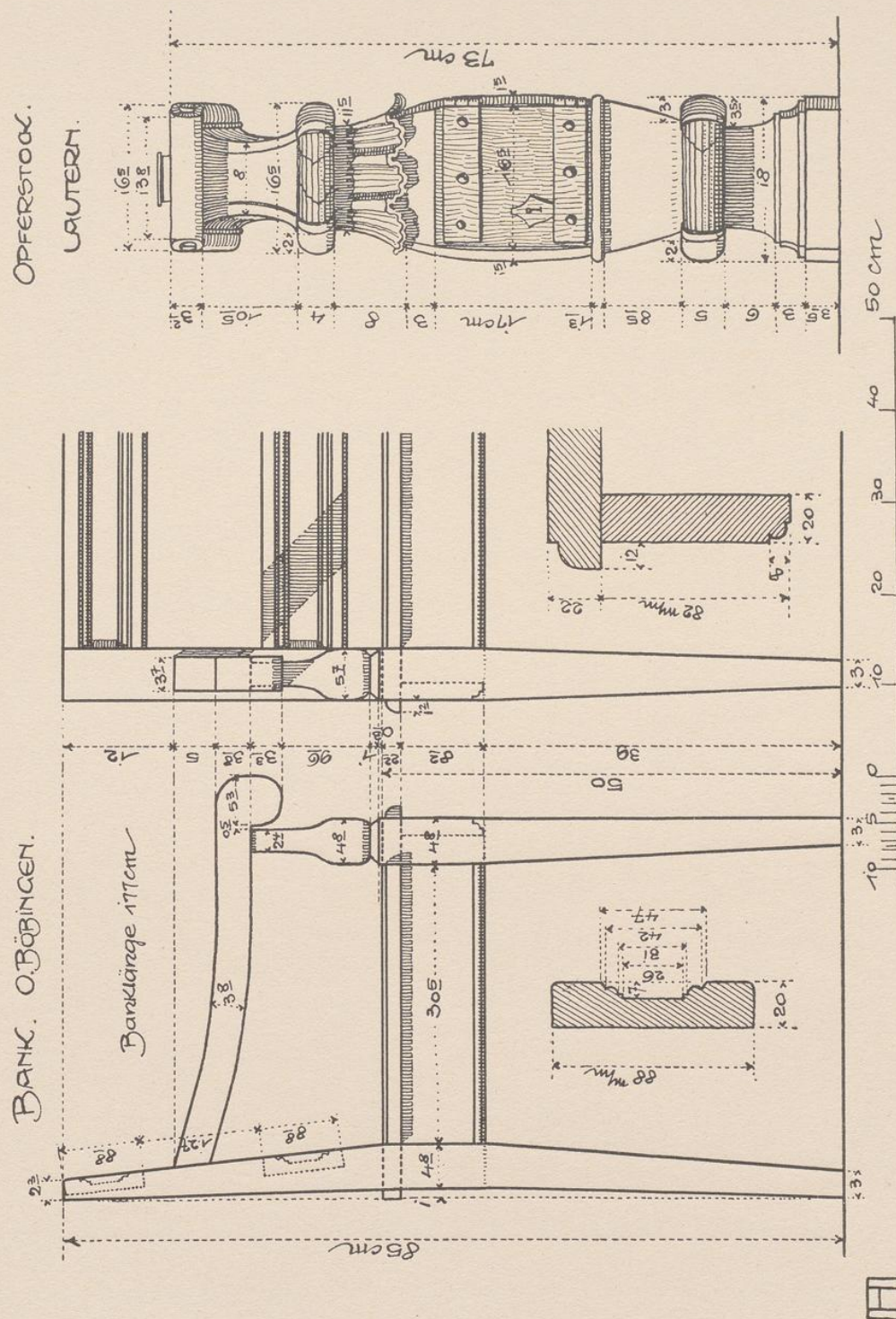
Bank. Opferstock mit eingebauter Eisenkassette.
