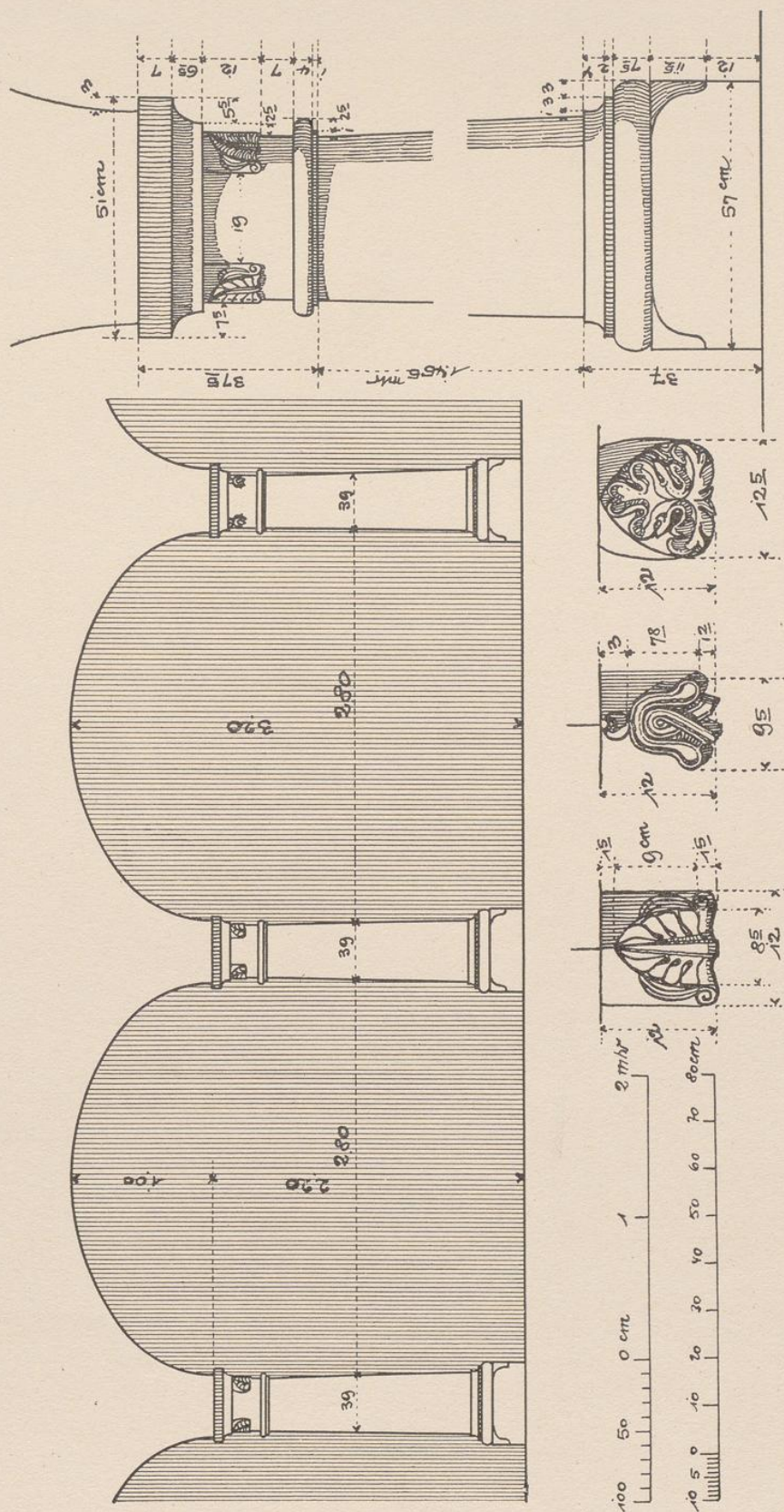
Arkaden mit Steinsäulen.
