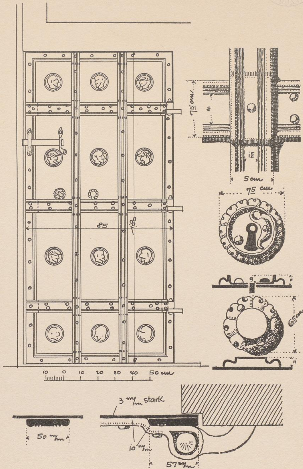
Eiserne Türe.
