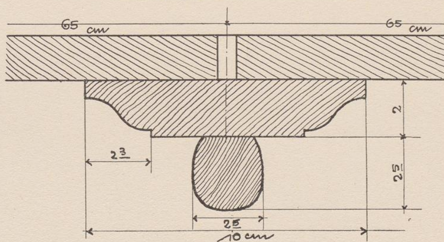
Hölzerne Rippendecke.
