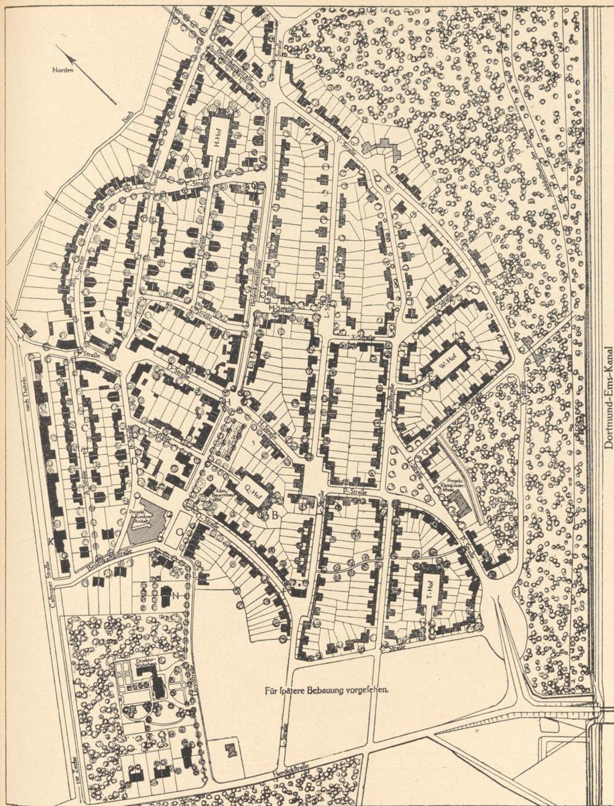
Siedlung Emscher Lippe - Lageplan.
