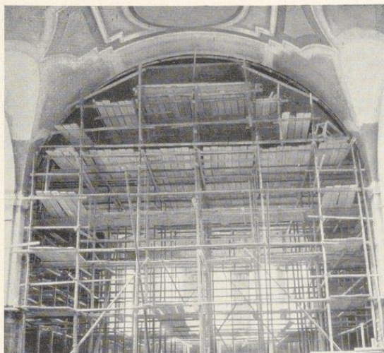
Bild 120. Hallengerüst aus Stangen, gebunden mit Hanfstricken. Köln
