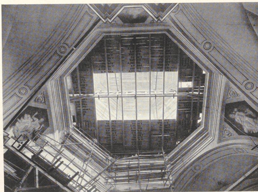
Bild 123. Die freitragende Rüstung von unten gesehen
