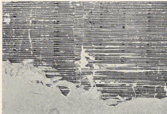
Bild 162. Richtige Stoßverbindung bei einfachen Rohrmatten
