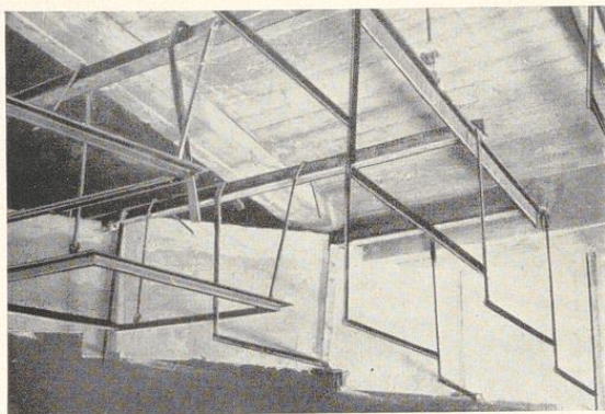
Bild 761. Entlüftungskanal aus Gipsplatten in einer Flacheisenkonstruktion aus Zürich
