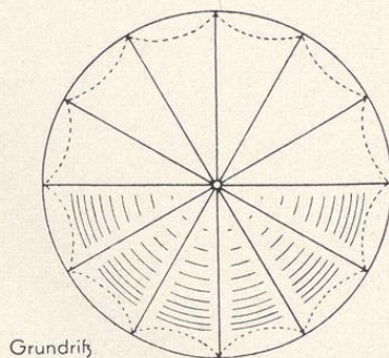
Schirmgewölbe mit Segmentbogen Schirmgewölbe mit Halbkreisbogen Schirmgewölbe mit Korbogen
