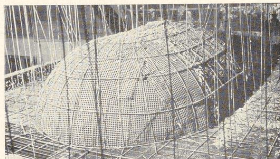
Bild 908. Das Gewölbe mit Staußziegelgewebe fertig ausgespannt, von oben gesehen
