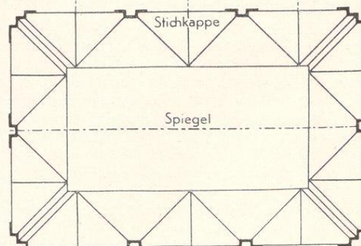
Spiegelgewölbe mit Stichkappen
