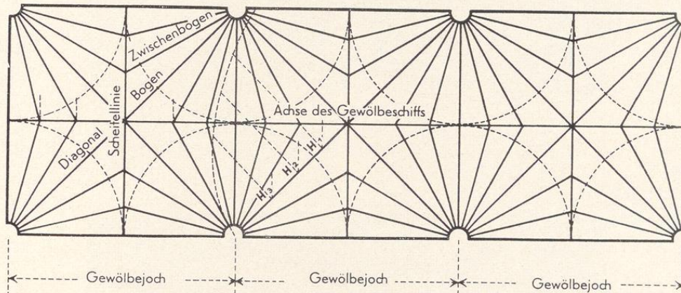
Fächergewölbe mit Spitzbogen und ebenem, gebustem Scheitel
