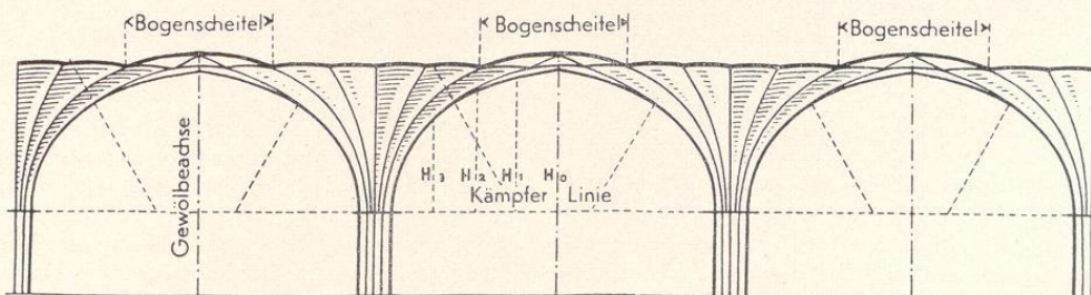
Bild 961. Die Konstruktionen der Fächer- und Trichtergewölbe
