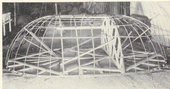
Bild 904. Rundeisengerippe eines kleinen Muldengewölbes von oben gesehen
