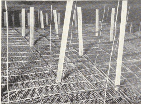
Bild 889. Rückseite des Rabitz-Tonnengewölbes von Bild 880. Gut ausgeführte Absteifung der Rundeisenbügel mit Latten
