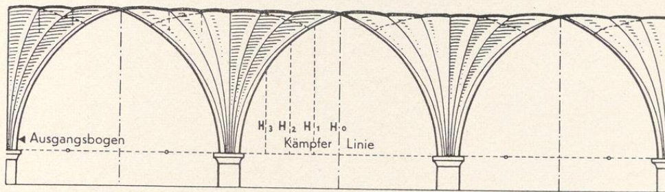
Fächergewölbe mit Spitzbogen und ebenem, gebustem Scheitel
