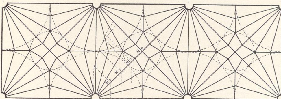
Fächergewölbe mit Korbbogen und Sternfigur im Scheitel
