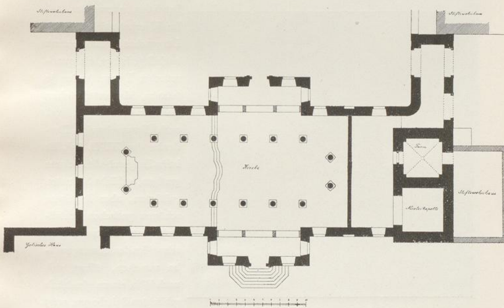
37. Steterburg, Grundriß der Kirche.
