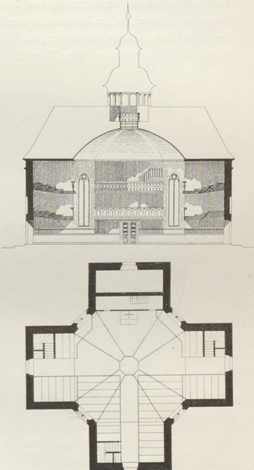
22. Kissenbrück, Querschnitt und Grundriß der Kirche.
