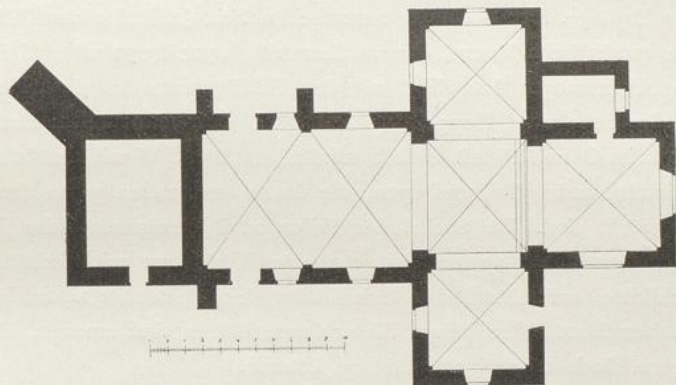
26. Salzdahlum, Grundriß der Kirche.
