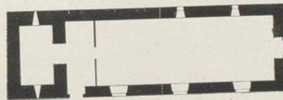
52. Volzum, Grundriß der Kirche.
