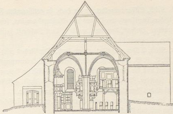
133. Stegelitz. Kirche. Querschnitt
