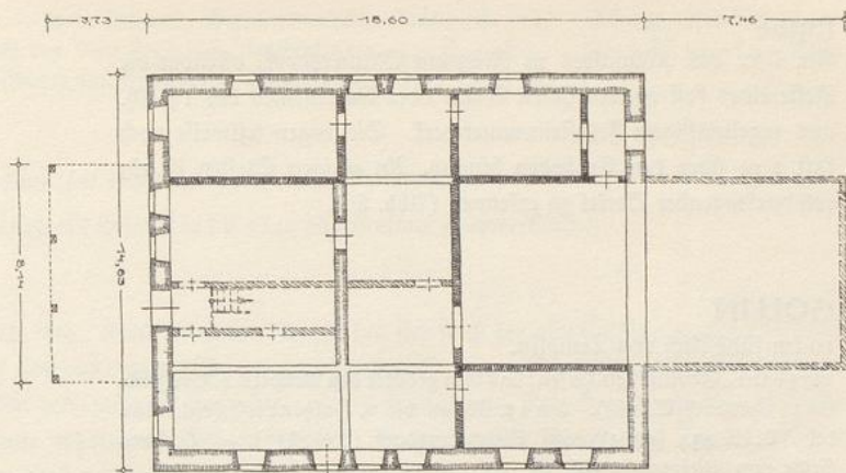
79. Gerswalde. Laubenhaus. Grundriß
