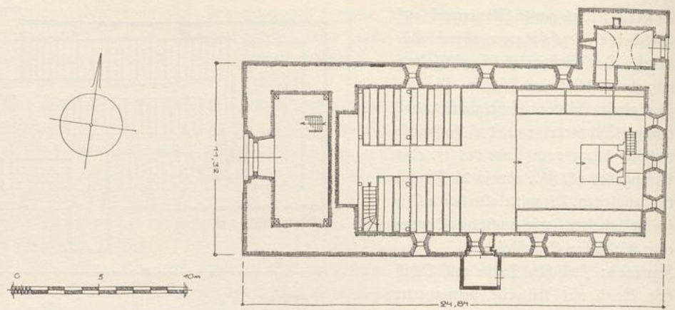
135. Strehlow. Kirche. Grundriß
