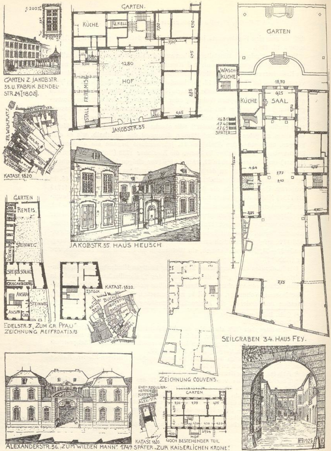
Abb. 26: Häuser mit Straßenhof.
