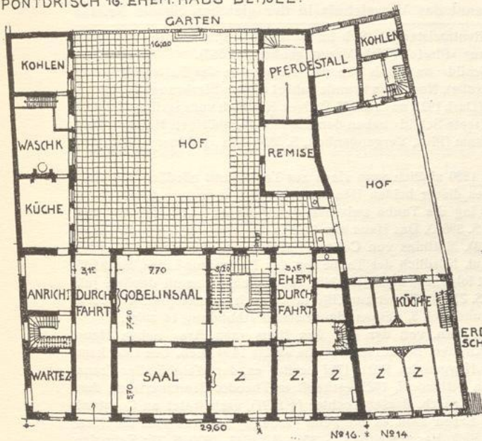
PONTDRISCH 16. EHEM. HAUS BEISEL.
