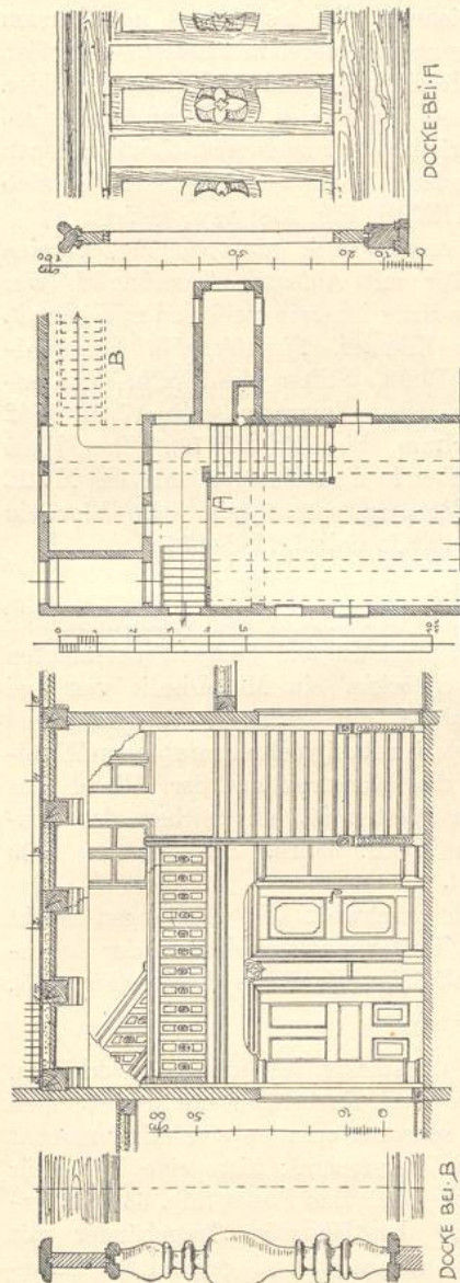
Fig. 334. Wollenweberstraße 12. Diele. Grundriß, Schnitt und Einzelheiten.
