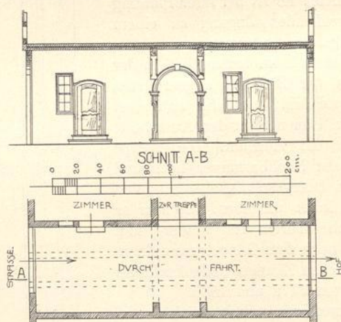
Fig. 272. Langer Hagen 53. Diele (Durchfahrt). Grundriß und Schnitt.
