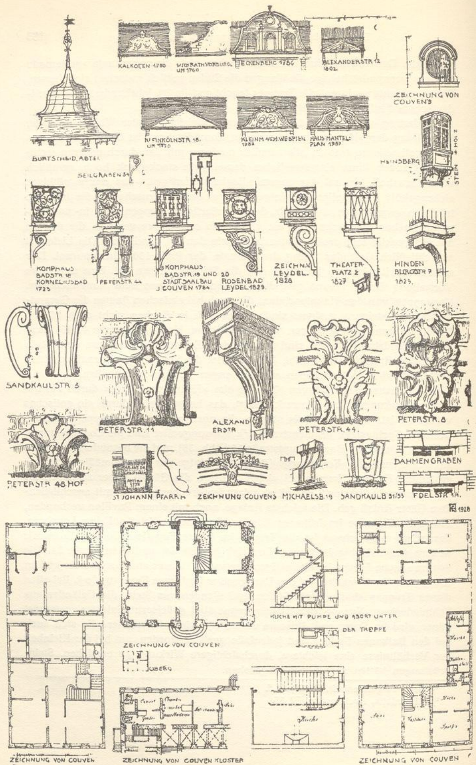
Abb. 65: Einzelheiten von Couven-Bauten.
