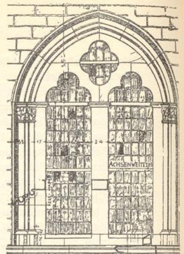
FISCHMARKT 3 GRASHAUS [I. ARCHIV] 1267 1:50
