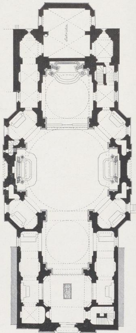
508. 509. Klosterkirche Rott am Inn, Längenschnitt, Grundriß, 1759—1763.
