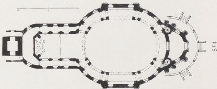
514. 515. Wallfahrtskirche Wies (Oberbaiern), Grundriß und Galerie im Chor, 1746.
