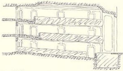
Abb. 974. Längsschnitt
