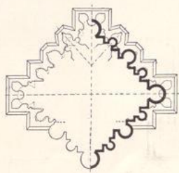
7. Straßburger Münster, Langhaus, vollendet 1275.
