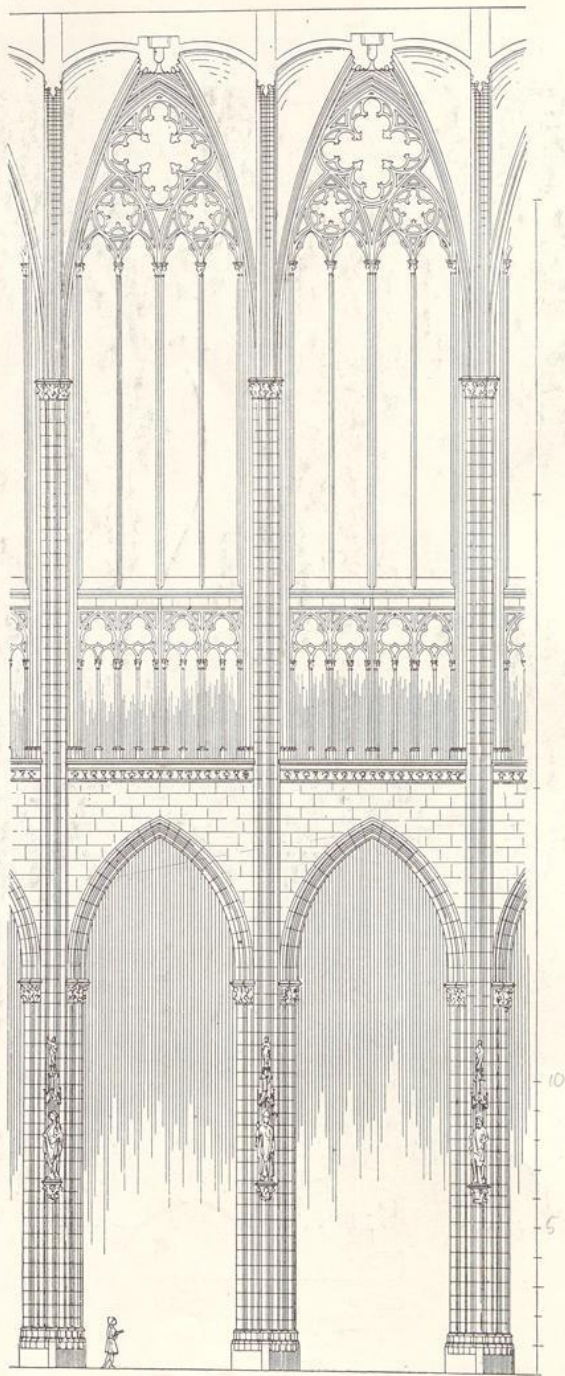
8. Kölner Dom, System des Langhauses.
