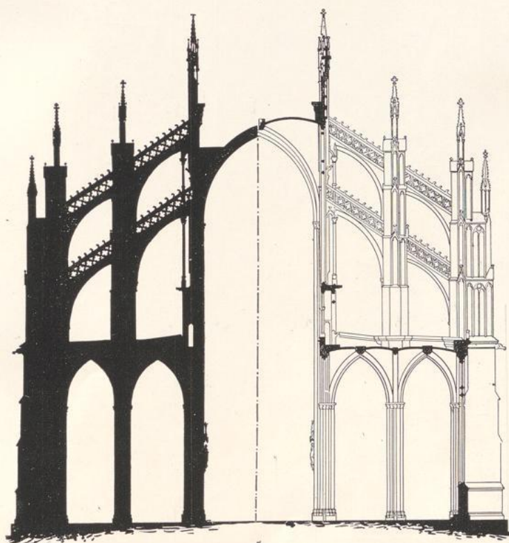
4. Straßburger Münster, Querschnitt. 5. Kölner Dom, Querschnitt.
