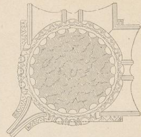
7. Grundriss des ionischen Eckkapitäls.
