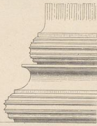
4. Säulenbasis. Von der Nordhalle des Erechtheion.
