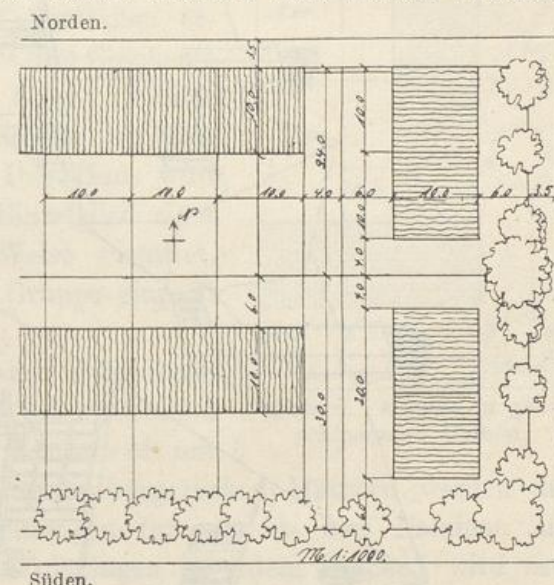
Abb. 2. Einseitig angebaute — Doppelhäuser — und eingebaute Reihenhäuser.
